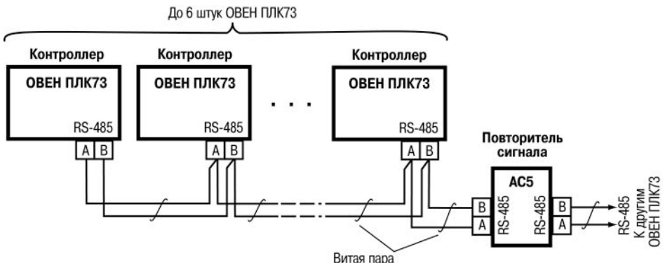
Рисунок 6.3 – Пример схемы подключений в сеть более 6-ти ОВЕН ПЛК73 (АС5 – повторитель сигнала разработки ОВЕН)
