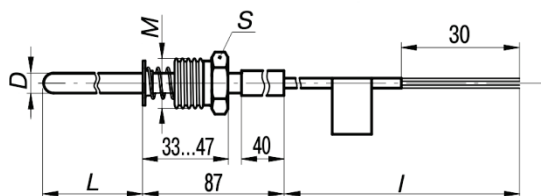
Рисунок A.6 – Конструктивные исполнения 124, 134 и 144
