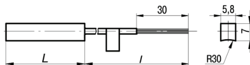
Рисунок A.10 – Конструктивное исполнение 224
