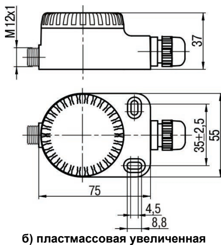
Рисунок В.3 – Конструктивные исполнения коммутационных головок для ОВЕН ДТС 125
