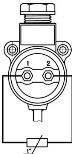
Рисунок Д.4 – Схемы подключения проводников к клеммам пластмассовых коммутационных головок датчиков типа ДТС 125 с одним ЧЭ
