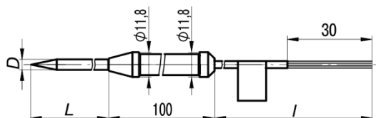
Рисунок A.8 – Конструктивные исполнения 164, 174 и 184
