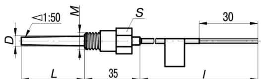
Рисунок A.9 – Конструктивное исполнение 204
