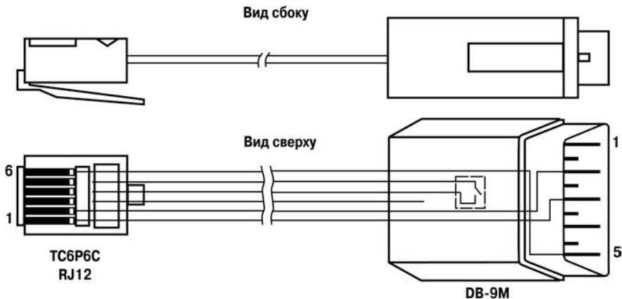
Рисунок Г.3 – Схема кабеля KS3 «ПЛК-Модем»
