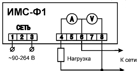
Рисунок Б.1 – Схема подключения прибора
