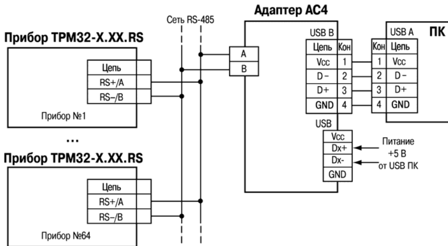
Рисунок В.5 – Схема подключения ОБЕН TPM32-Щ4.01.RS и ОБЕН TPM32-Щ4.03.RS к адаптеру сети ОБЕН AC4
