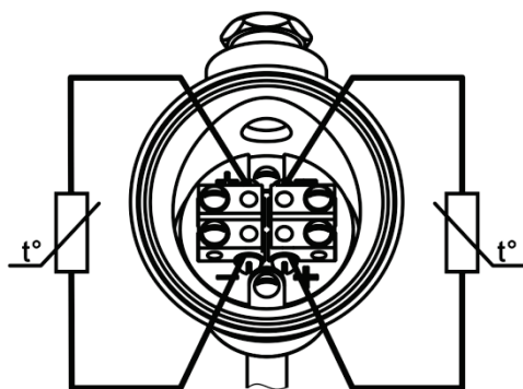
а) двухпроводная
