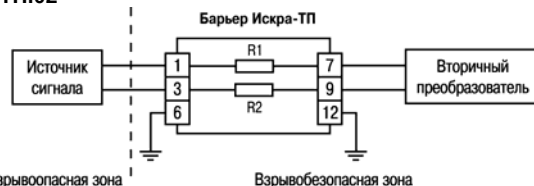
Рисунок 2 – Схема подключения барьера, R1=R2=110 \text{ Ом} \pm 5 \%
