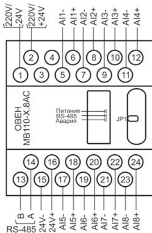
Рисунок Б.1 – Общий вид прибора
