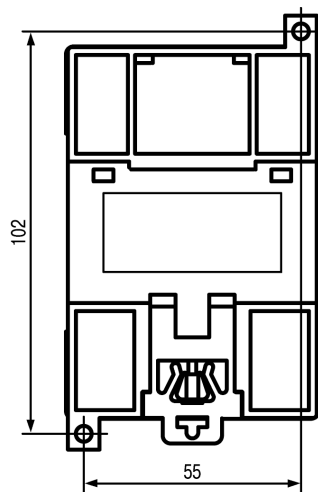
Рисунок А.2 – Установочные размеры
