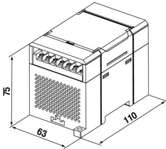
Рисунок А.1 – Габаритный чертеж прибора ОВЕН МВ110-Х.8АС
