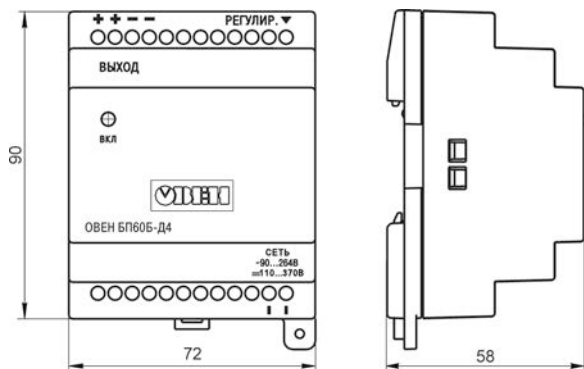
Рисунок 3.1 – Габаритные размеры блока
