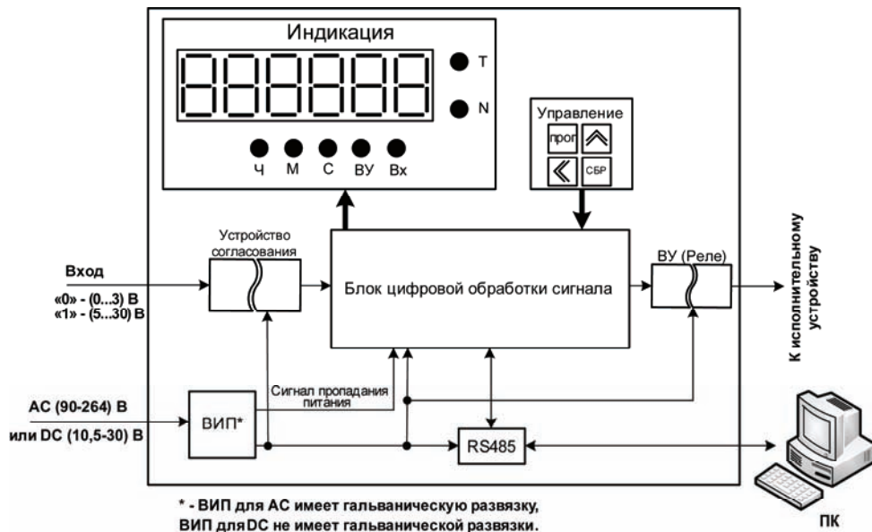
Рисунок 3.1 – Функциональная схема
