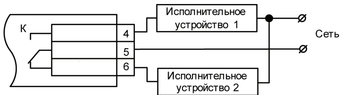
Рисунок Б.2 – Схема подключения нагрузки к ВУ типа Р
