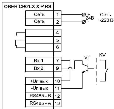
Рисунок Б.1 – Подключение датчиков имеющих на выходе транзистор n-р-п типа с открытым коллекторным входом или подключение к входу коммутационных устройств:
