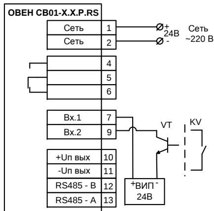
Рисунок Б.1 – Подключение датчиков имеющих на выходе транзистор n-р-п типа с открытым коллекторным входом или подключение к входу коммутационных устройств:
