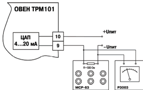
Рисунок Ж.5 – Подключение ВУ2 вида И
