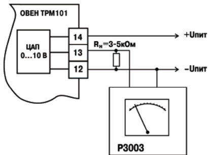
Рисунок Ж.6 – Подключение ВУ1 вида У
