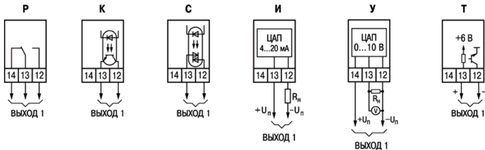
Рисунок Б.2 – Схемы подключения различных исполнений ВУ1
