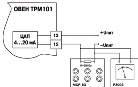
Рисунок Ж.4 – Подключение ВУ1 вида И
