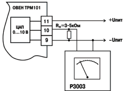
Рисунок Ж.7 – Подключение ВУ2 вида У
