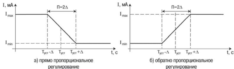
Рисунок 3.13 – Принцип формирования управляющего тока П - регулятора
