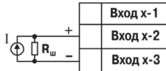
R_n = (50,000 \pm 0,025) \text{ Ом} Рисунок Б.12 – Схема подключения активного датчика с выходом в виде тока от 0 до 5 мА или от 0 до 20 мА или от 4 до 20 мА
