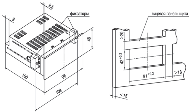
Рисунок А.4 – Прибор щитового крепления Щ2
