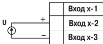
Рисунок Б.11 – Схема подключения активного датчика с выходом в виде напряжения от минус 50 до 50 мВ или от 0 до 1 В
