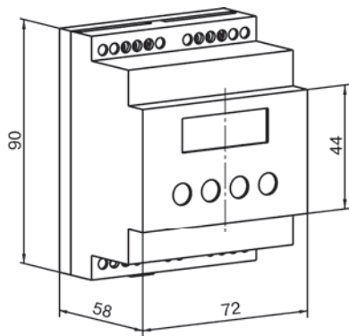
Рисунок А.5 – Прибор с креплением на DIN-рейку
