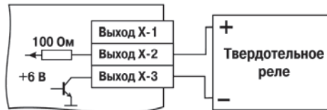
Рисунок Б.6 – Схема подключения нагрузки к ВУ вида И
