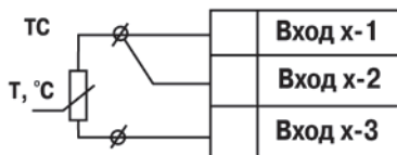
Рисунок Б.9 – Схема подключения термопреобразователя сопротивления
