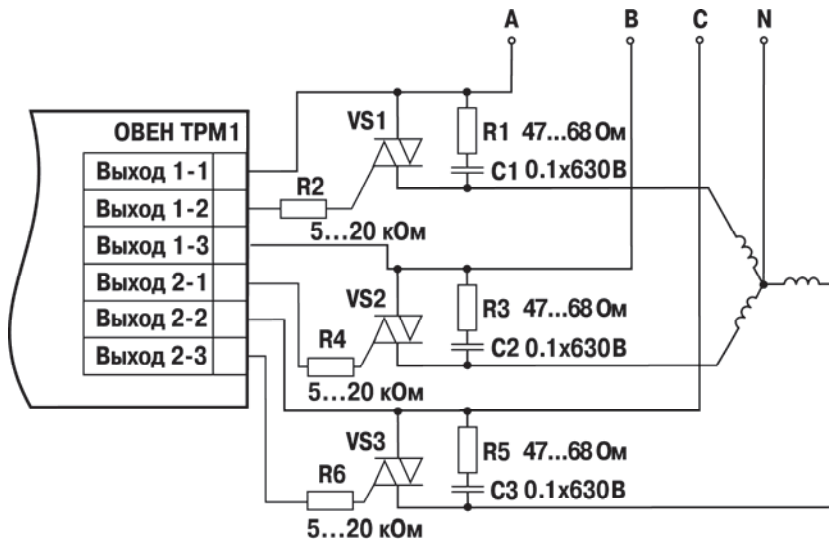
Рисунок Б.5 – Схема подключения трех симисторных оптопар (для ОВЕН ТРМ1-Х.У.С3)
