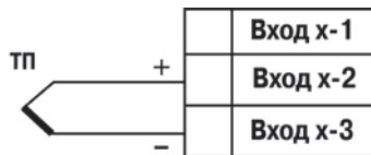
Рисунок Б.10 – Схема подключения преобразователя термоэлектрического
