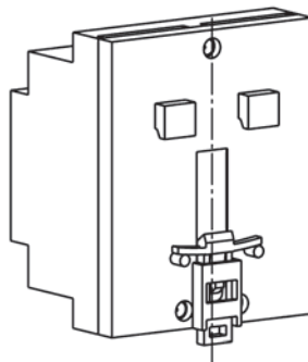
Рисунок А.5 – Прибор с креплением на DIN-рейку
