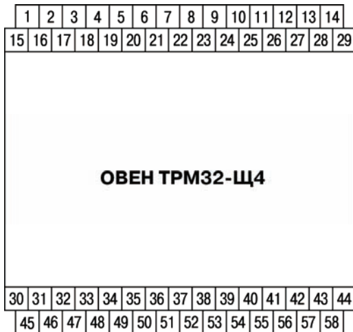
Рисунок В.1 – Схема расположения клеммных соединителей ОВЕН ТРМ32-Щ4
