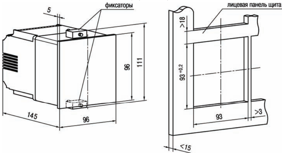
Рисунок Б.1 – Габаритные и установочные размеры ОВЕН ТРМ32-Щ4
