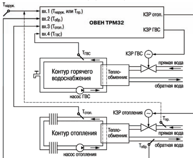
Рисунок А.1 – Схема системы отопления и ГВС
