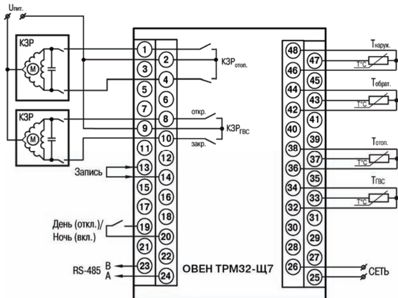
Рисунок В.3 – Схема подключения ОВЕН ТРМ32-Щ7
