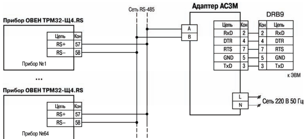
Рисунок В.4 – Схема подключения ОВЕН ТРМ32-Щ4.01.РС и ОВЕН ТРМ32-Щ4.03.РС к адаптеру сети ОВЕН АС3М
