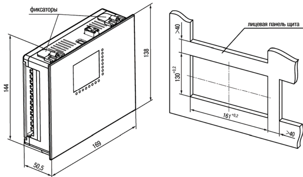
Рисунок Б.2 – Габаритные и установочные размеры ОВЕН ТРМ32-Щ7
