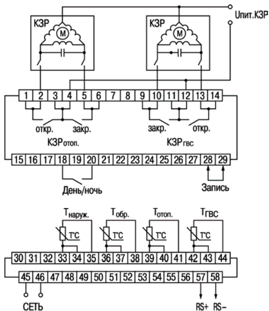
Рисунок В.2 – Схема подключения ОВЕН ТРМ32-Щ4
