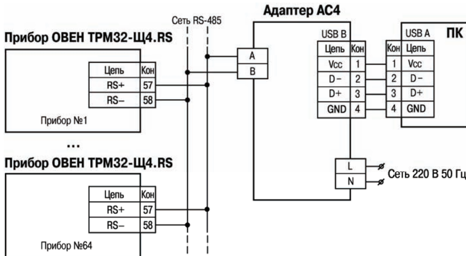
Рисунок В.5 – Схема подключения ОВЕН ТРМ32-Щ4.01.RS и ОВЕН ТРМ32-Щ4.03.RS к адаптеру сети ОВЕН АС4
