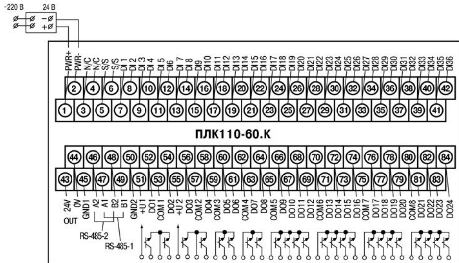
Рисунок Б.2 – Схема расположения и назначение клемм на ПЛК110-24.60.K. Схема для ПЛК110-220.60.K – аналогична
