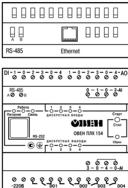
Рисунок 4.1 – Внешний вид контроллера
