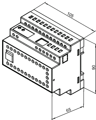
Рисунок А.1 – Габаритные размеры ОВЕН ПЛК154
