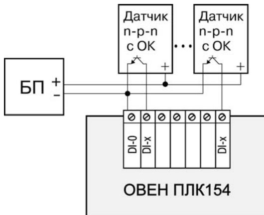
Рисунок Б.5 – Схема подключения к ОВЕН ПЛК154 дискретных датчиков с полупроводниковым выходным каскадом
