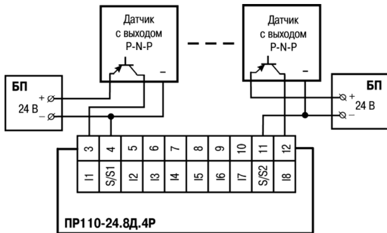
Рисунок Б.4 – Схема подключения к ПР110-24.8Д.4Р трехпроводных дискретных датчиков, имеющих выходной транзистор p-n-p -типа с открытым коллектором
