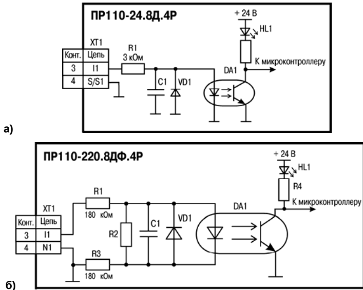
Рисунок Б.5 – Электрическая схема входов для разных исполнений прибора (схемы других входов идентичны приведенным, но для входов I5–I8 общим является контакт 11)
