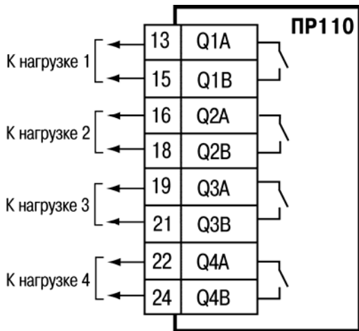
Рисунок Б.2 – Подключение нагрузок к выходным контактам реле
