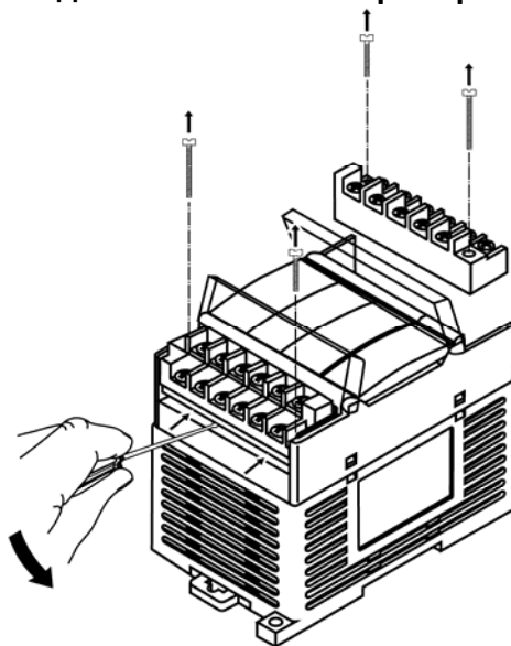
Рисунок В.1 – Отделение съемных частей клемм на корпусе ПР110
