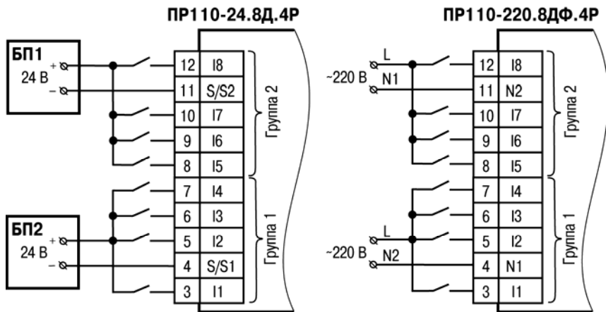
Рисунок Б.3 – Подключение к ПР110 дискретных датчиков с выходом типа «сухой контакт»
