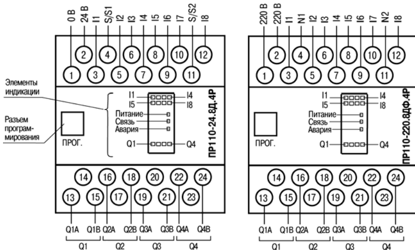
Рисунок Б.1 – Расположение контактов и элементов индикации в приборах PR110
