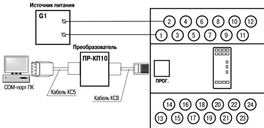
Рисунок Б.6 – Схема подключения ПР110 к ПК (через преобразователь ПР-КП10), G1 – источник питания с номинальным напряжением, зависящим от исполнения прибора
