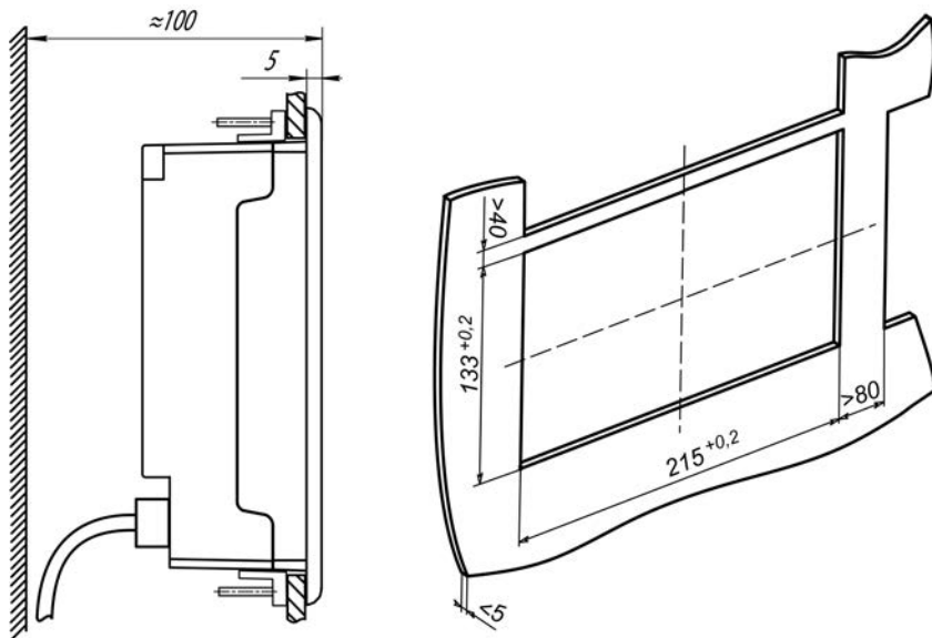
Рисунок А.2 – Установочные размеры СПК207
