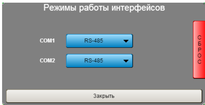
Рисунок Д.7 - Конфигуратор СПК107/110. Режимы работы интерфейсов
