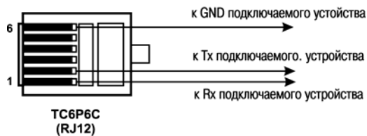
Вид сверху
