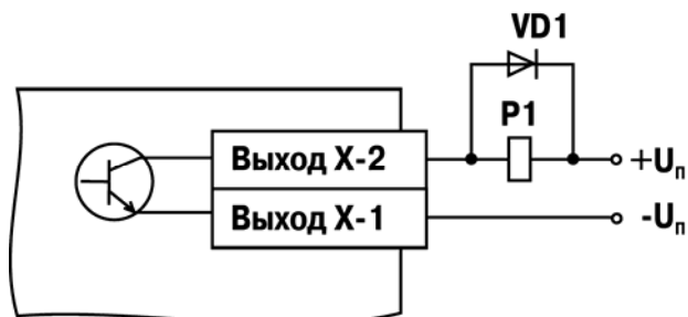
Рисунок Б.9 – Схема подключения нагрузки к ВУ типа К
