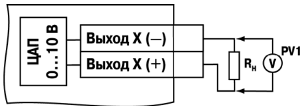
Рисунок Б.14 – Схема подключения нагрузки к ВУ типа У. R_H > 2 \text{ кОм}
