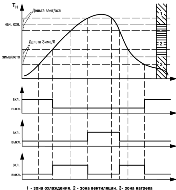
1 - зона охлаждения, 2 - зона вентиляции, 3- зона нагрева Рисунок 5.2 – Условия перехода между режимами «Нагрев»-«Вентиляц»-«Охлаждение»
