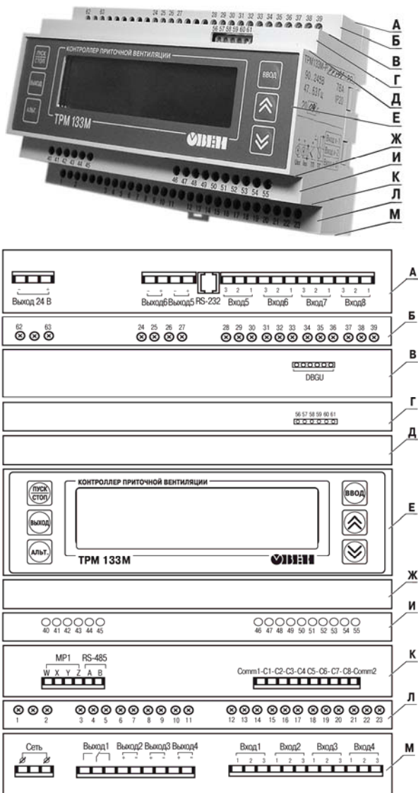
Рисунок 3.1 – Прибор TPM133M-02: внешние связи, элементы индикации и управления
