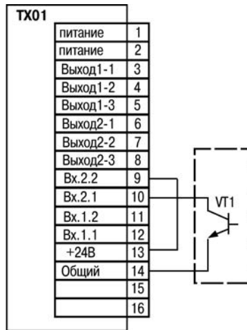
Рисунок Б.2 – Подключение пассивных датчиков, имеющих на выходе транзистор n-p-n типа с открытым коллекторным входом: а) при работе датчика от внешнего источника питания; б) при работе датчика от питающего напряжения прибора
