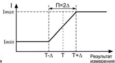
б) прямо пропорциональное регулирование
