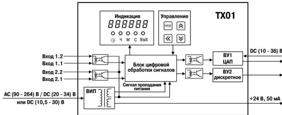
Рисунок 3.1 – Функциональная схема
