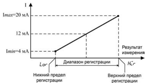
Рисунок 4.4 – Принцип формирования выходного сигнала ВУ в режиме регистратора для приборов с ВУ типа И
