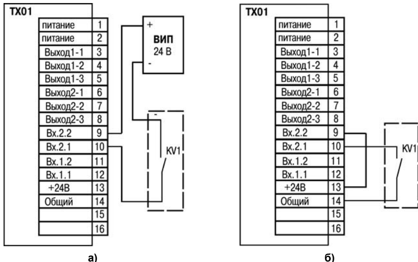
Рисунок Б.1 – Подключение к входу коммутационных устройств: а) при работе датчика от внешнего источника питания; б) при работе датчика от внутреннего источника питания
