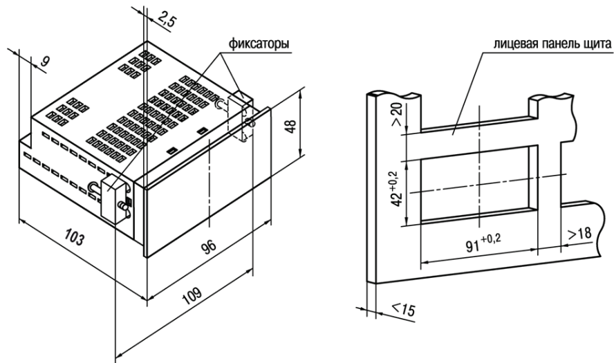
Рисунок А.3 – Прибор щитового крепления в корпусе типа Щ2
