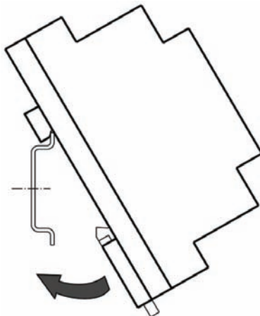
Рисунок 28 – Монтаж прибора с креплением на DIN-рейку
