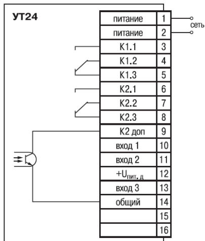
Рисунок Б.1 – Схема подключения прибора модификации УТ24-Х.Р
