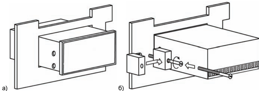
Рисунок 27 – Монтаж прибора настенного исполнения
