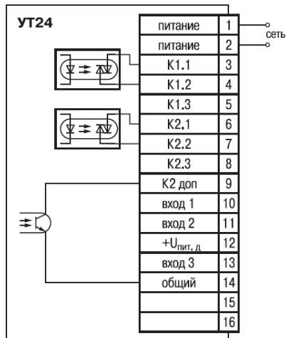
Рисунок Б.2 – Схема подключения прибора модификации УТ24-Х.С
