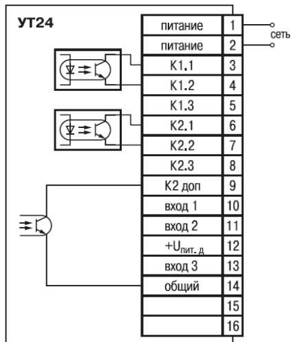
Рисунок Б.3 – Схема подключения прибора модификации УТ24-Х.К
