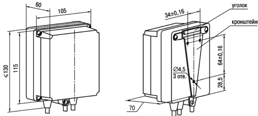
Рисунок А.1 – Прибор настенного крепления в корпусе типа Н
