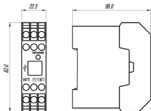
Рисунок 2 – Внешний вид преобразователя
