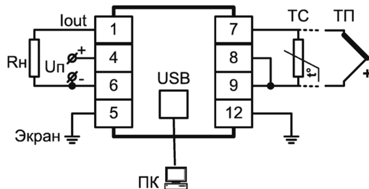
Рисунок 3 – Клеммные соединители преобразователя и схема подключения датчиков
