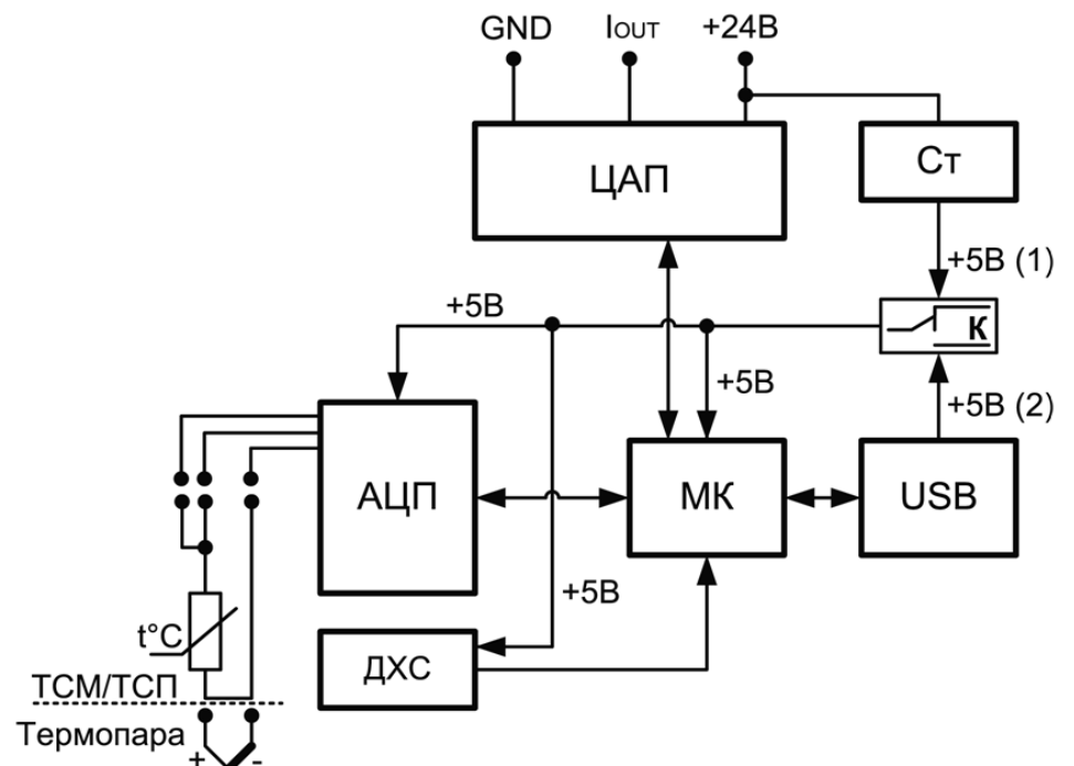
Рисунок 1 – Структурная схема преобразователя
