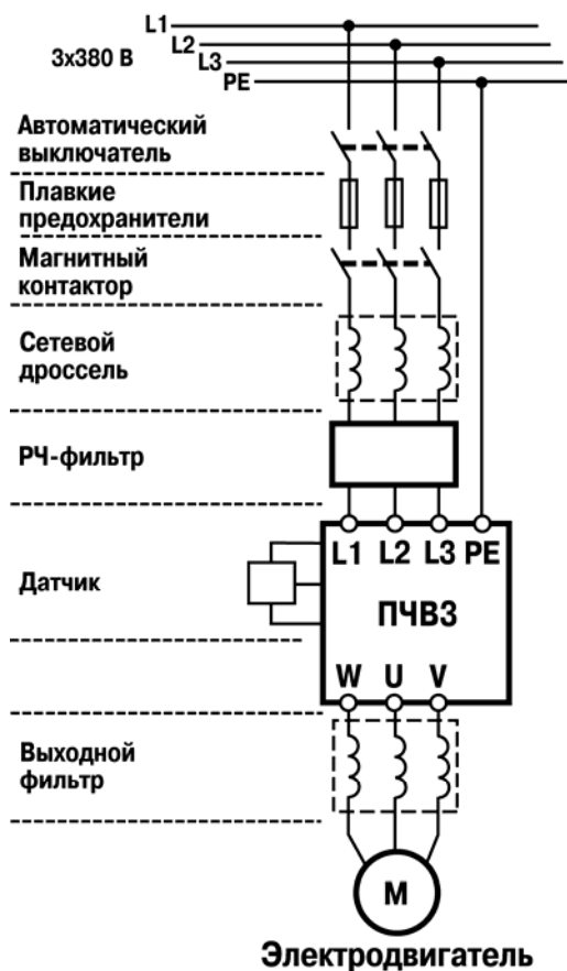
Рисунок 2.1 - Рекомендуемая структурная схема привода ПЧВЗ
