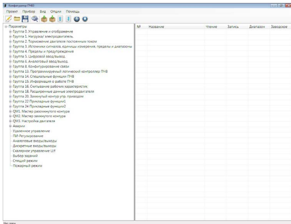
Рисунок 6.1 – Внешний вид окна программы «Конфигуратор ПЧВЗ»
