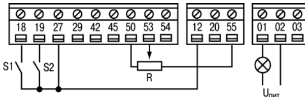
Рисунок 4.1 - Схема внешних подключений ПЧВЗ
