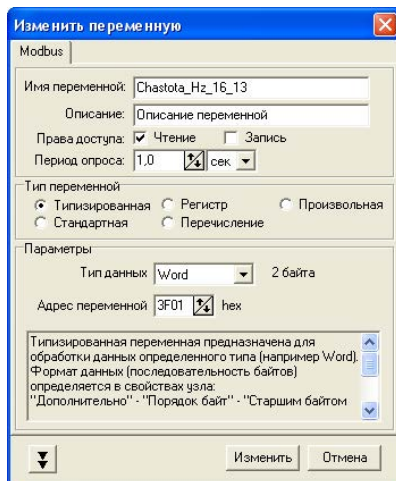
Рисунок 5.13 - Настройка переменной ПЧВЗ 16-13 Частота, Гц для отображения в ОРС
