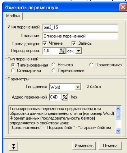
Рисунок 5.14 - Настройка переменной ПЧВЗ 3-15 Источник задания 1 для отображения в ОРС
