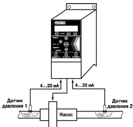
Рисунок 4.6 - Схема установки
