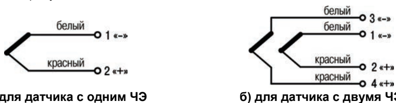
Рисунок 6.1 – Схемы внутренних соединений проводов датчиков типа ОВЕН ДТФХ ХХ4
