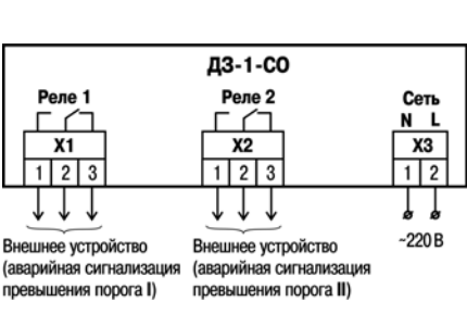
Рисунок 5.2 – Функциональное назначение клемм прибора
