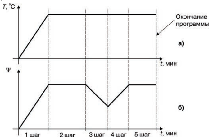
Рисунок 6.2 – Определение общего числа шагов в программе:
