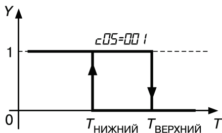
Рисунок 3.15 – Компаратор срабатывает по нижней уставке:
