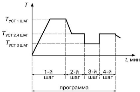
Рисунок 3.26 – Пример графика программы
