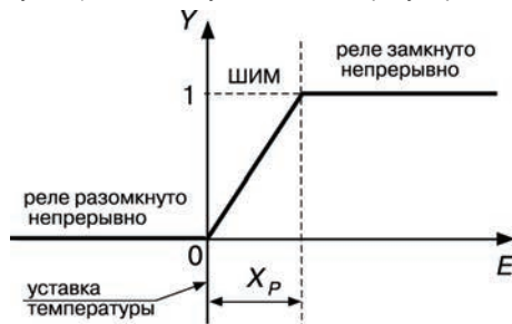
Рисунок 3.7 – П-закон регулирования
