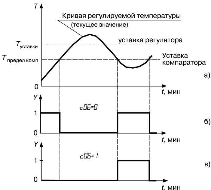
Рисунок 3.18 – Блокировка срабатывания компаратора до первого достижения уставки
