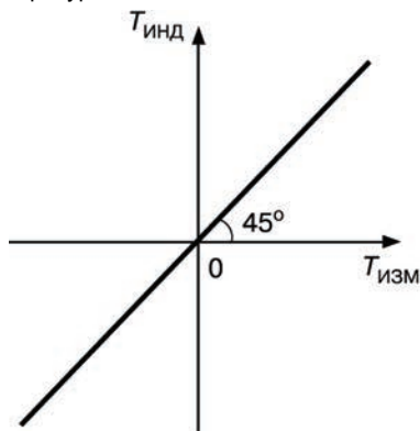
Рисунок 3.3 – Характеристика исправного датчика
