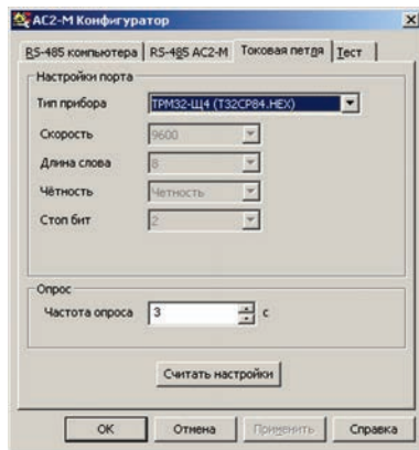
Рисунок Л.4 – Конфигуратор AC2-M. Вкладка "Токовая петля"
