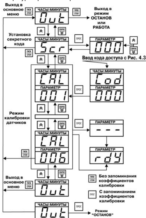
Рисунок 4.6 – Схема, поясняющая программирование на уровне L4
