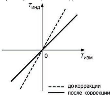
Рисунок 3.6 – Коррекция "наклон характеристики"
