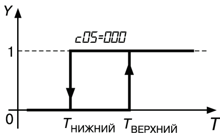
Рисунок 3.14 – Компаратор срабатывает по верхней уставке:
