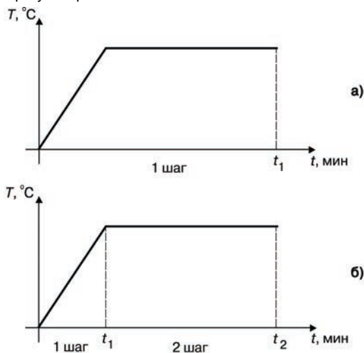
Рисунок 6.1 – Пример разбиения технологического режима на шаги:
