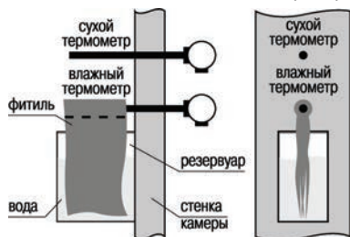
Рисунок Е.1 – Крепление датчиков температуры перпендикулярно стенке камеры
