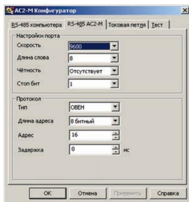
Рисунок Л.3 – Конфигуратор AC2-M. Вкладка "RS-485 AC2-M"
