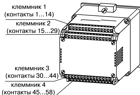
Рисунок Б.3 – Вид прибора сзади
