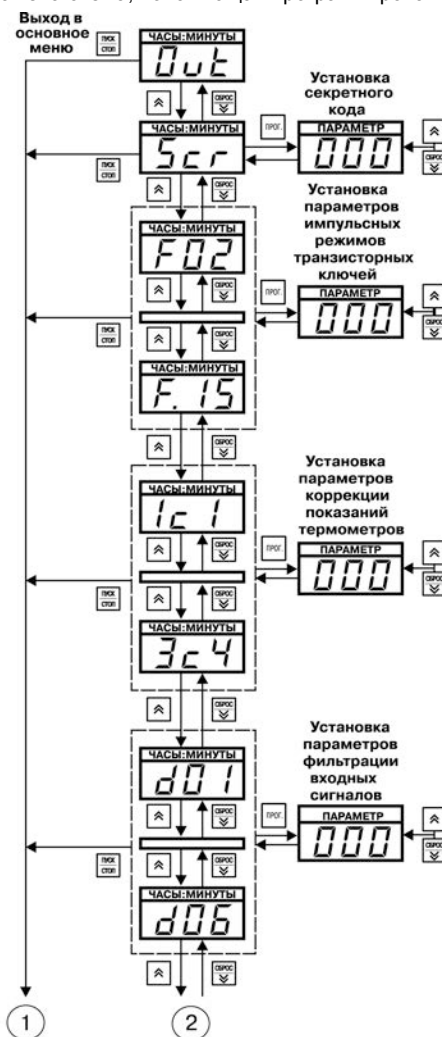
Рисунок 4.3 – Схема, поясняющая программирование на уровне L2
