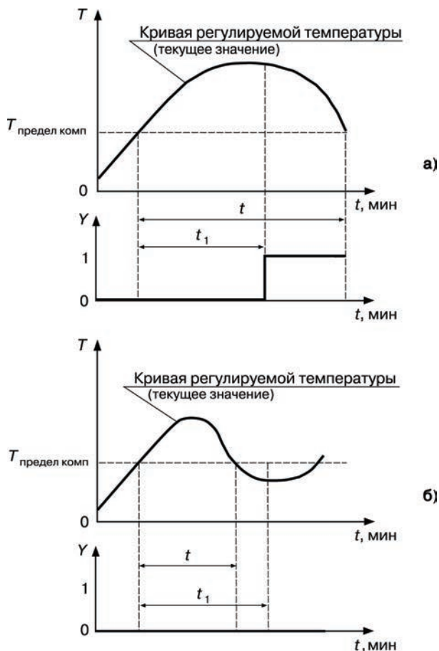
Рисунок 3.19 – Задержка срабатывания компаратора:
