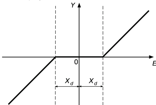
Рисунок 3.13 – Зона нечувствительности для исполнительного устройства типа «нагреватель-холодильник» или «задвижка»
