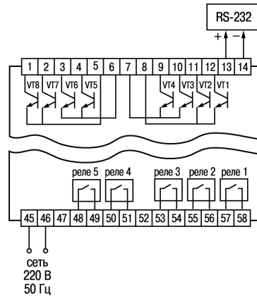
Рисунок Б.2 – Подключение транзисторных ключей и выходных устройств
