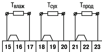
Рисунок В.2– Соединение датчиков по двухпроводной схеме
