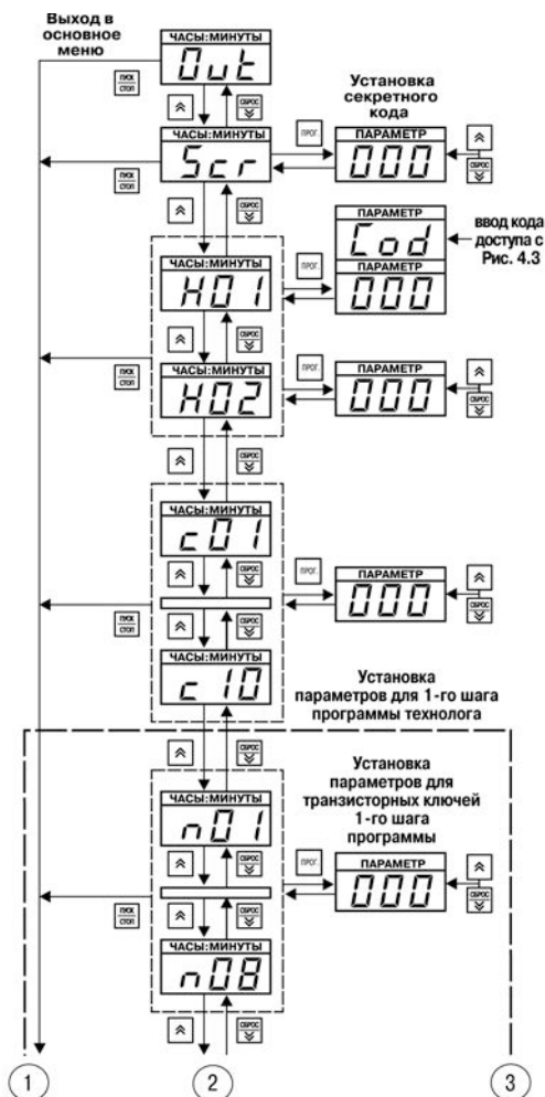
Рисунок 4.4 – Схема, поясняющая программирование на уровне L1
