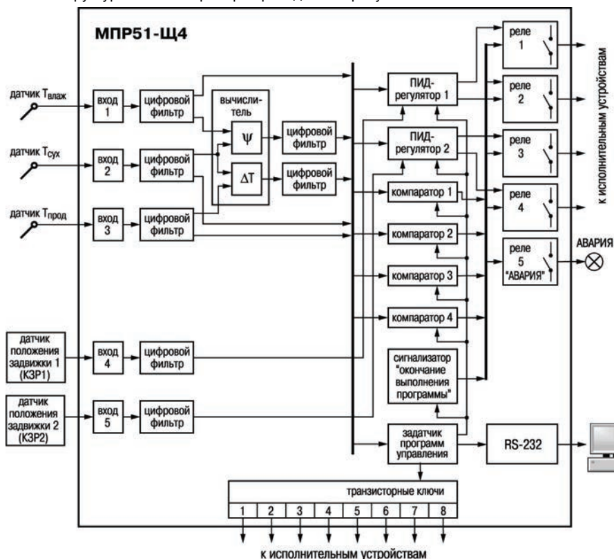
Рисунок 3.1 – Структурная схема прибора
