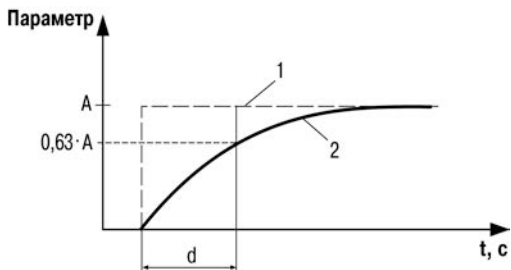
Рисунок 3.2 – Принцип действия фильтра
