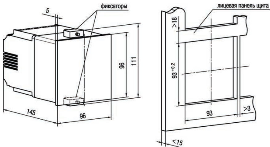
Рисунок А.1 – Габаритный чертеж
