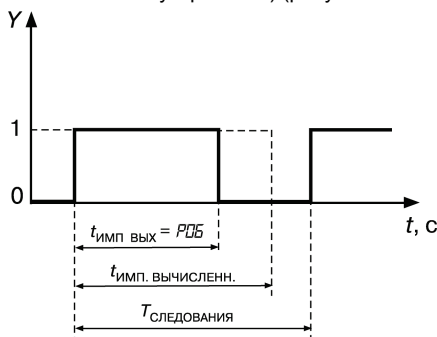
Рисунок 3.10 – Ограничение максимальной мощности. Временная диаграмма
