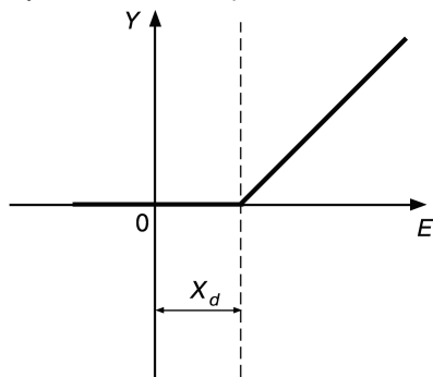
Рисунок 3.12 – Зона нечувствительности для исполнительного устройства типа «нагреватель»
