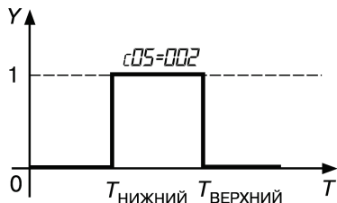
Рисунок 3.16 – Компаратор срабатывает внутри установленных пределов
