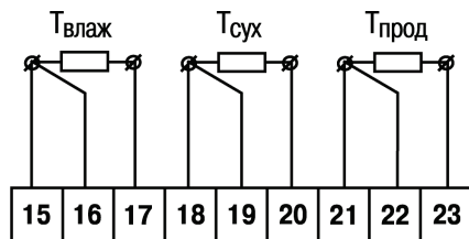
Рисунок В.1– Соединение датчиков по трехпроводной схеме
