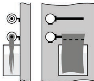
Рисунок Е.2 – Крепление датчиков температуры параллельно стенке камеры
