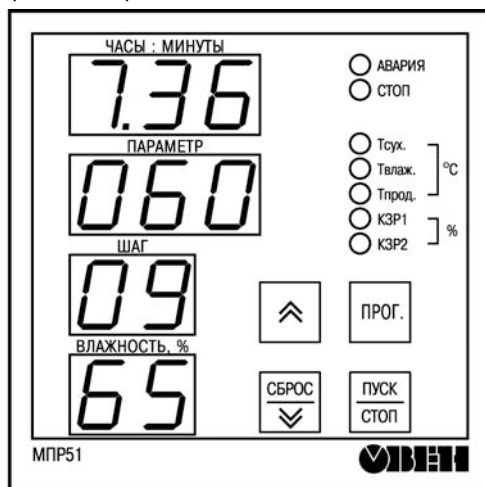
Рисунок 3.27 – Лицевая панель прибора
