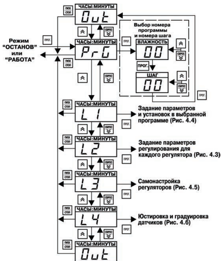
Рисунок 4.2 – Основное меню режима «ПРОГРАММИРОВАНИЕ»
