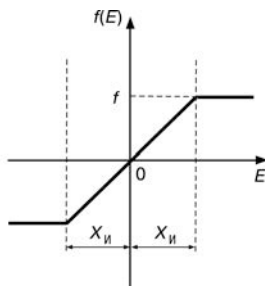
Рисунок 3.9 – Ограничение интегральной составляющей при помощи X_{и}
