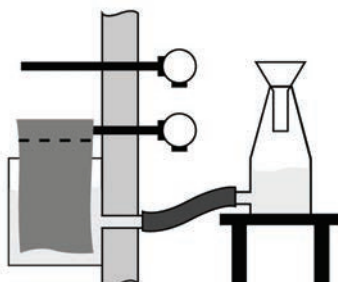
Рисунок Е.4 – Конструкция резервуара для воды, не требующая входа в камеру
