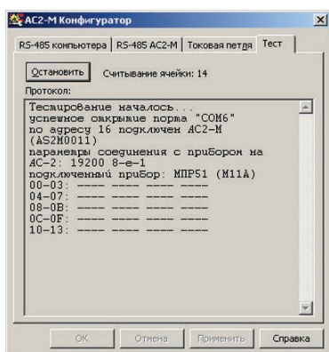
Рисунок Л.5 – Конфигуратор AC2-M.
