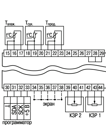
Рисунок Б.1 – Подключение измерительных датчиков и датчиков положения задвижек
