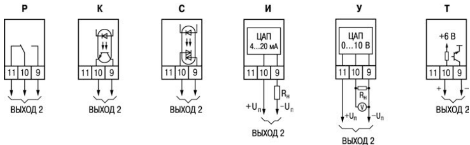
Рисунок Б.3 – Схемы подключения различных исполнений ВУ2
