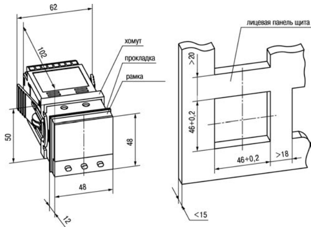
Рисунок А.1 – Крепление с помощью крепежного хомута
