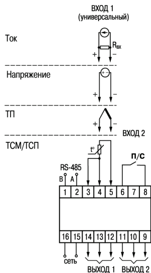
Рисунок Б.1 – Общая схема подключения
