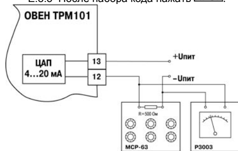
Рисунок Е.4 – Подключение ВУ1 вида «И»
