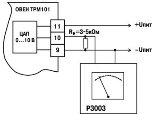
Рисунок Е.7 – Подключение ВУ2 вида «У»
