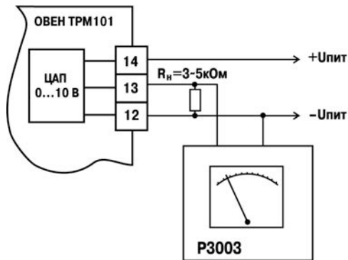
Рисунок Е.6 – Подключение ВУ1 вида «У»
