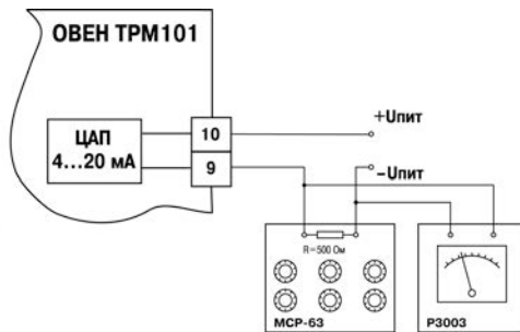
Рисунок Е.5 – Подключение ВУ2 вида «И»
