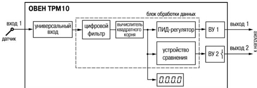
Рисунок 3.1 – Структурная схема прибора
