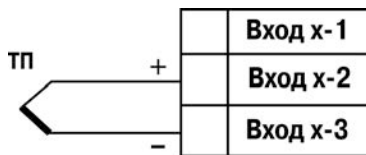
Рисунок Б.10 – Схема подключения преобразователя термоэлектрического
