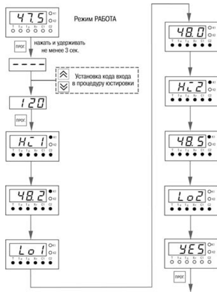
Рисунок Ж.2 – Последовательность запуска и индикации АНР для ОВЕН ТРМ10-Щ1.Р
