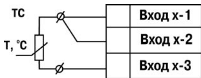
Рисунок Б.9 – Схема подключения термопреобразователя сопротивления
