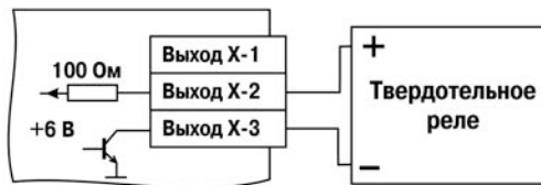
Рисунок Б.8 – Схема подключения нагрузки к ВУ вида Т
