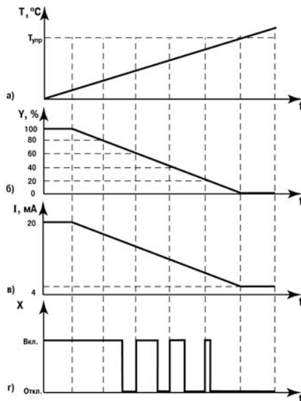
Рисунок 3.11 – Принцип управления в режиме «Нагреватель»: а) изменение температуры объекта; б) сигнал на выходе регулятора; в) сигнал на аналоговом выходе И; г) сигнал на дискретном выходе типа Р
