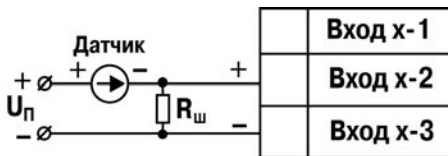
Рисунок Б.12 – Схема подключения активного датчика с выходом в виде тока от 0 до 5 мА или от 0 до 20 мА или от 4 до 20 мА
