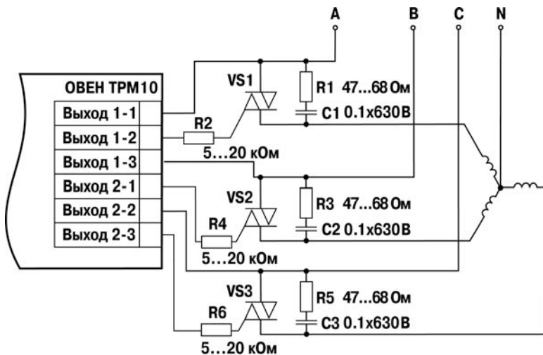
Рисунок Б.5 – Схема подключения трех симисторных оптопар
