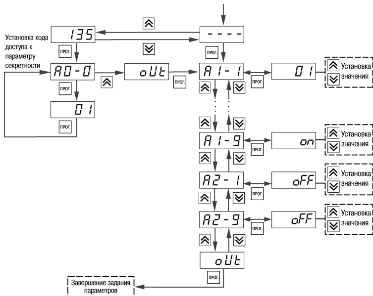
Рисунок 6.3 – Последовательность работы с прибором на втором уровне программирования (для группы параметров А)
