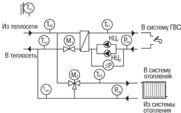
Рисунок Л.3 – Два независимых контура ГВС и отопление с циркуляционными насосами для контура ГВС
