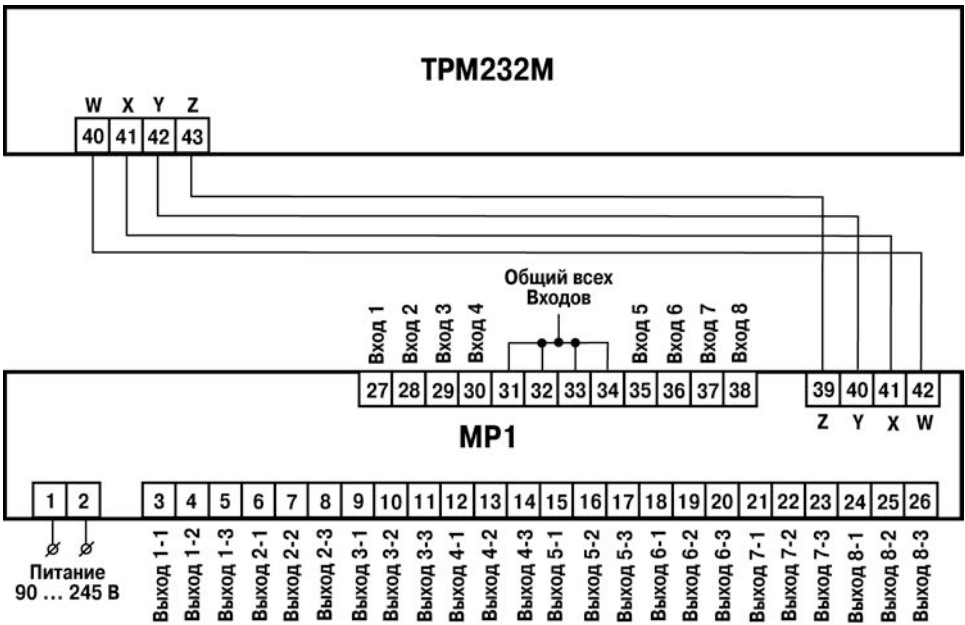
Рисунок Б.1 – Схема подключения TPM232M и MP1
