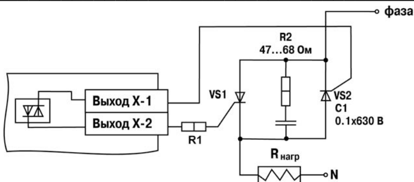
Рисунок Б.11 – Схема подключения нагрузки к ВУ типа С двух тиристорах, подключенных встречно-параллельно
