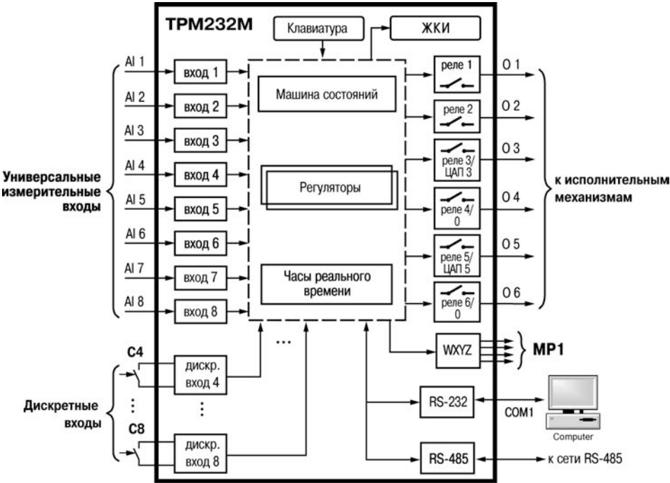
Рисунок 3.2 – Структурная схема прибора
