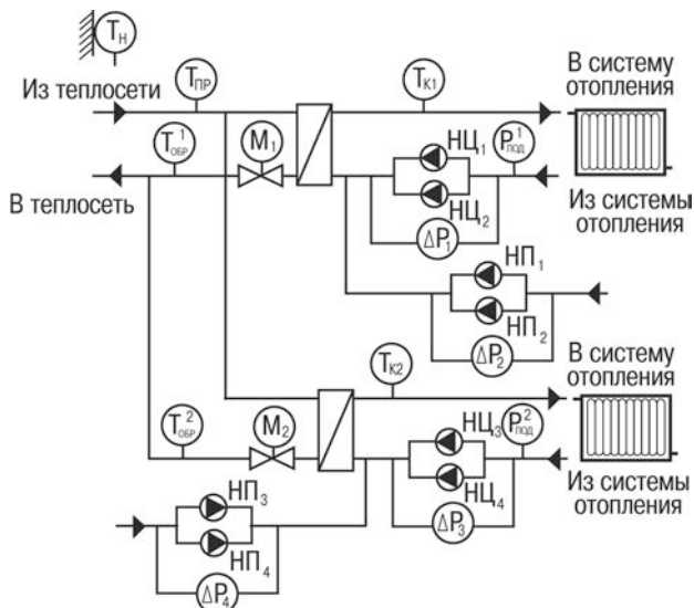
Рисунок Л.4 – Два независимых контура отопления с циркуляционными насосами и насосами подпитки
