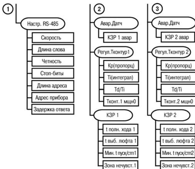
Рисунок И.1 – Главное меню прибора (продолжение)
