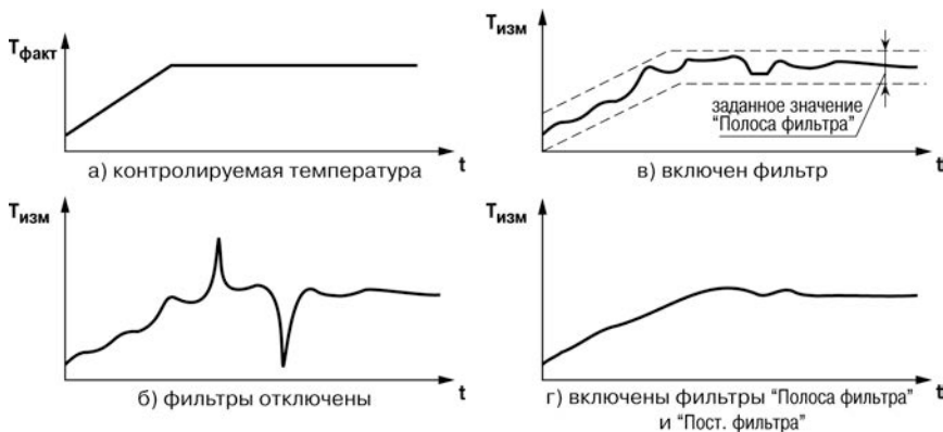
Рисунок 3.3 – Временные диаграммы работы цифровых фильтров показаний датчика
