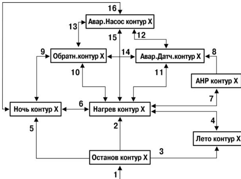
Рисунок 4.2 – Схема перехода между режимами контура
