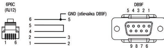
Рисунок Д.1 – Схема кабеля KC1
