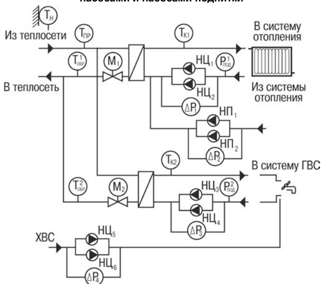
Рисунок Л.5 – Два независимых контура отопления и ГВС с насосами подпитки для контура отопления и насосами ХВС в контуре ГВС
