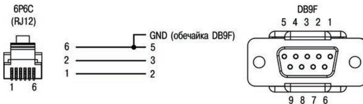
Рисунок Д.2 – Схема кабеля KC2
