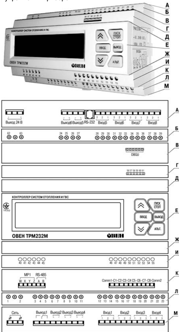
Рисунок 3.1 – Прибор TPM232M: клеммники, элементы индикации и управления
