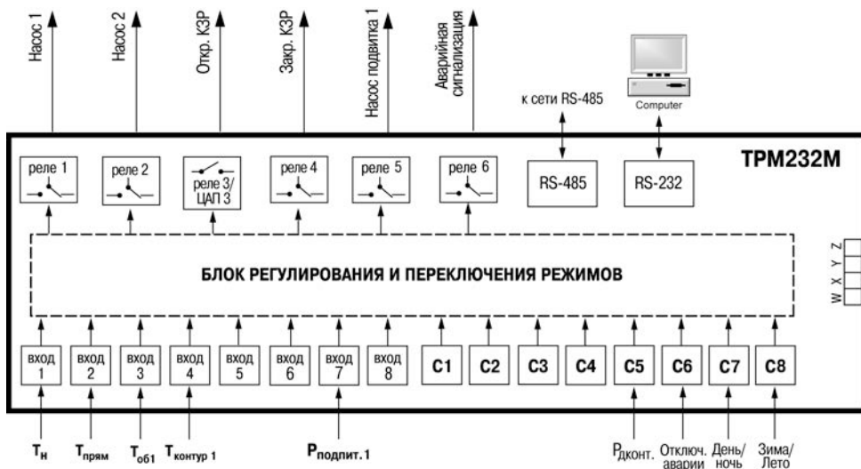
Рисунок 3.8 – Функциональная схема прибора, один контур
