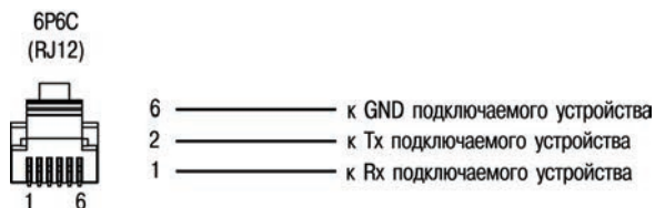
Рисунок Д.3 – Схема распайки соединительного кабеля для подключения к порту RS-232
