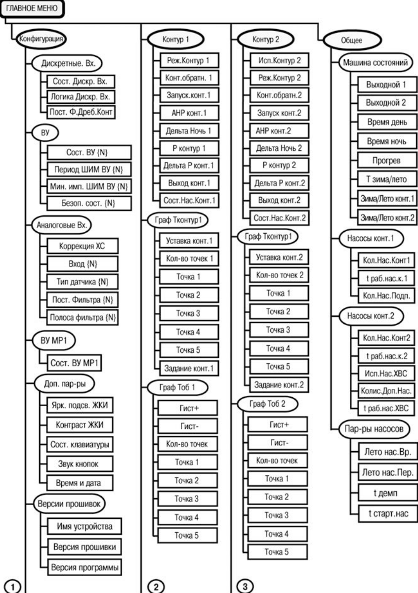
Рисунок И.1 – Главное меню прибора
