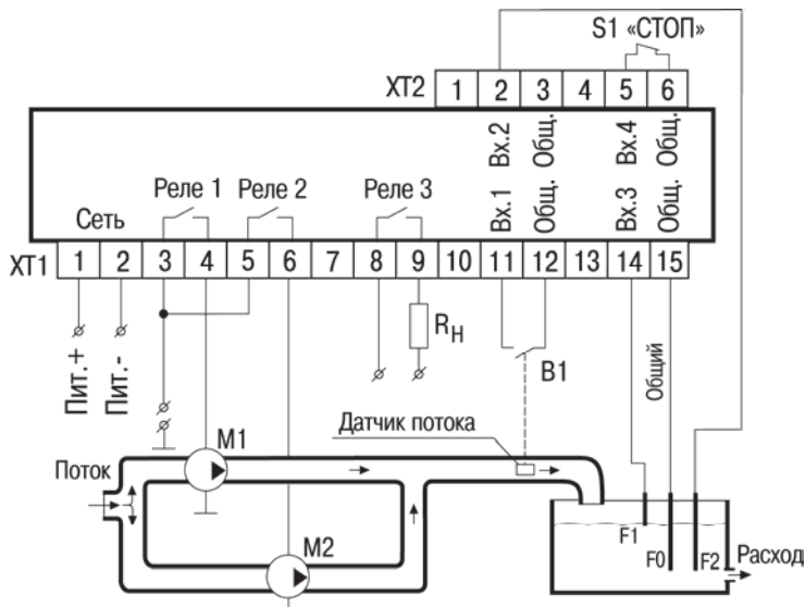
Рисунок В.8 – Схема подключения ОВЕН САУ-У-Н для выполнения алгоритма 12 M1 и M2 – насосы; R_H – сигнализатор аварии или дополнительный насос; B1 – датчик потока; F1, F2 – кондуктометрические датчики уровня
