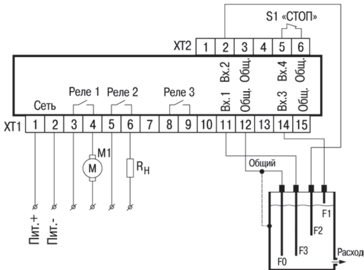
Рисунок В.1 – Схема подключения ОВЕН САУ-У-Н для выполнения алгоритма 01 М1 – исполнительное устройство (насос, электромотор, клапан или др.); R н – сигнализатор (звонок, сирена, лампа или блокирующий контактор); F1–F3 – кондуктометрические датчики уровня
