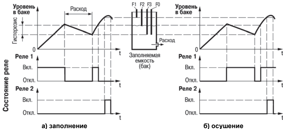
Рисунок В.2 – Графики, поясняющие работу прибора
