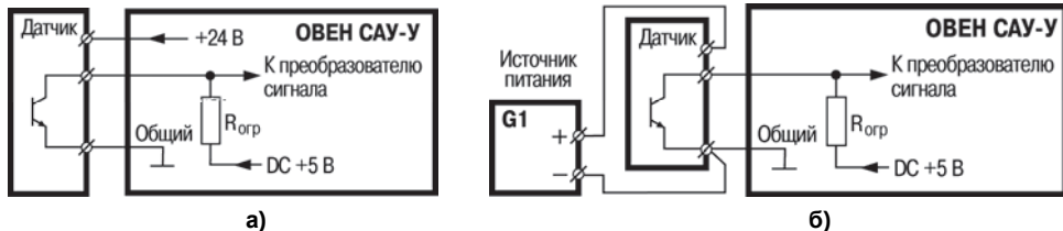
Рисунок 3.8 – Схема подключения датчиков с выходными ключами n-p-n типа: а) с питанием от прибора; б) с питанием от внешнего источника
