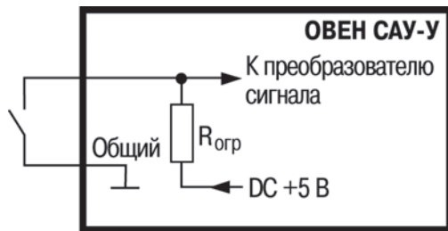
Рисунок 3.7 – Схема подключения механических контактных датчиков
