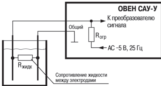
Рисунок 3.6 – Схема подключения кондуктометрического зонда
