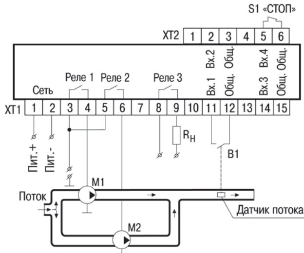
Рисунок В.6 – Схема подключения ОВЕН САУ-У-Н для выполнения алгоритма 11 М1 и М2 – насосы; R н – сигнализатор аварии или дополнительный насос; В1 – датчик потока
