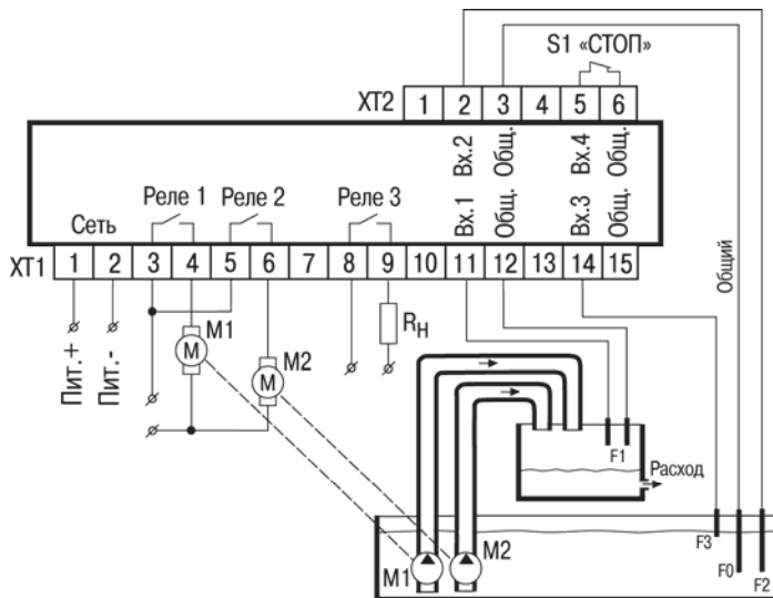
Рисунок В.14 – Схема подключения ОВЕН САУ-У-Н для выполнения алгоритма 18 M1 и M2 – насосы; F1–F3 – кондуктометрические датчики уровня; Rн – сигнализатор аварии (неисправность насоса)
