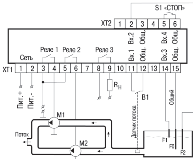
Рисунок В.12 – Схема подключения ОВЕН САУ-У-Н для выполнения алгоритма 16 М1 и М2 – насосы; R н – сигнализатор аварии или дополнительный насос; В1 – датчик потока; F1, F2 – кондуктометрические датчики уровня
