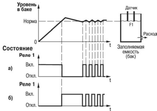
Рисунок В.5 – Графики, поясняющие работу прибора:
