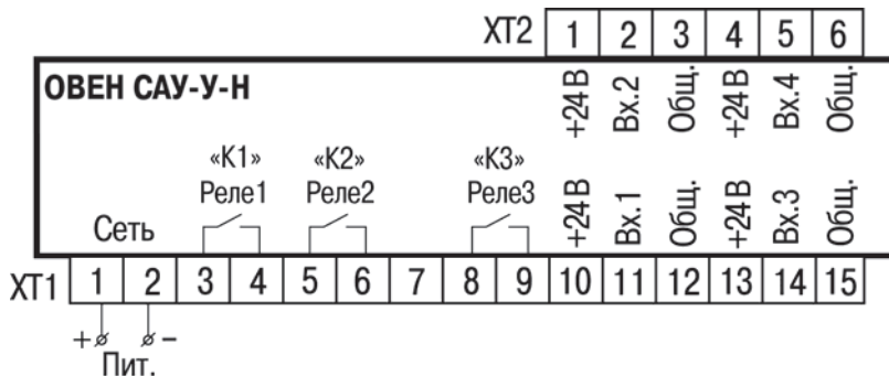
Рисунок Б.1 – Схема подключения ОВЕН САУ-У-Н
