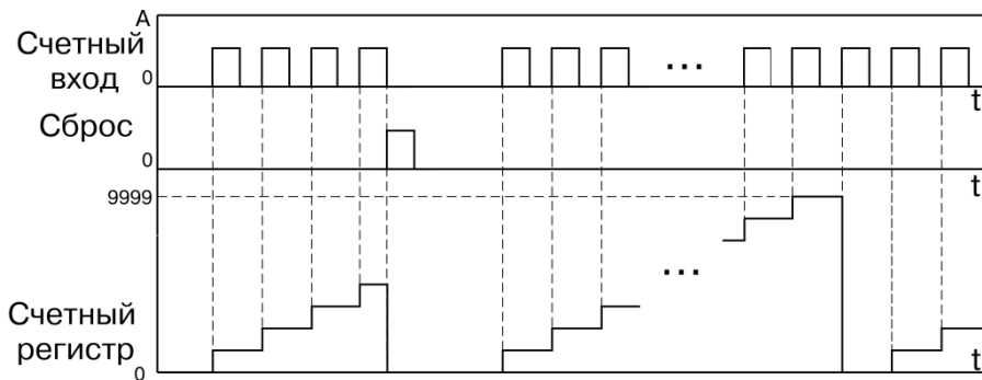
Рисунок 3.4 – Диаграмма работы прибора
