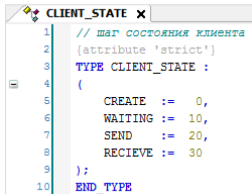
Рисунок 4.3.6 – Объявление перечисления CLIENT_STATE
