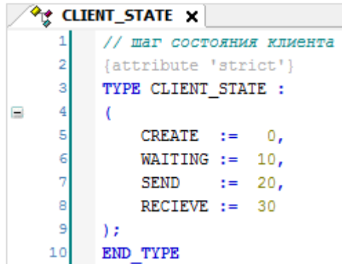
Рисунок 4.2.5 – Объявление перечисления CLIENT_STATE
