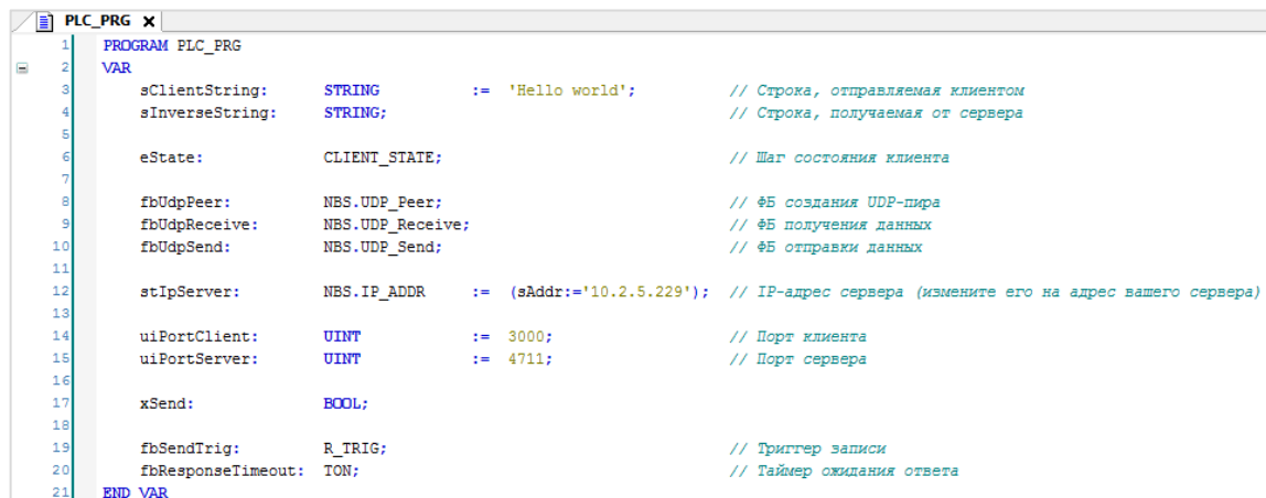
Рисунок 4.2.6 – Объявление переменных программы PLC_PRG
