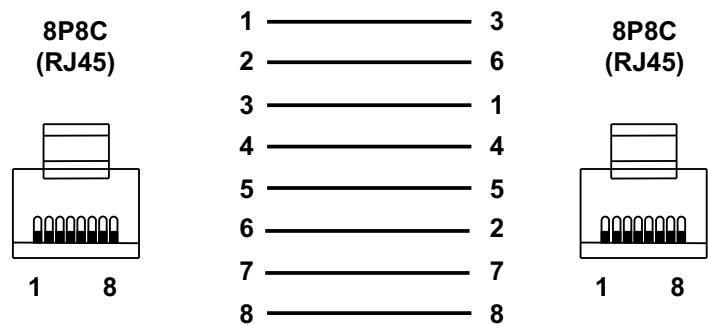
Рисунок 5.7 – Схема перекрестного кабеля для соединения прибора по сети Ethernet
