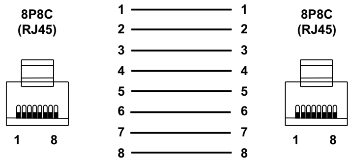
Рисунок 5.6 – Схема прямого кабеля для соединения прибора по сети Ethernet
