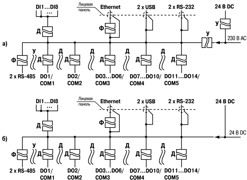
Рисунок 2.2 – Схема электрической прочности изоляции ПЛК110-220.Х.К(М02) (а) и ПЛК110-24.Х.К(М02) (б)
