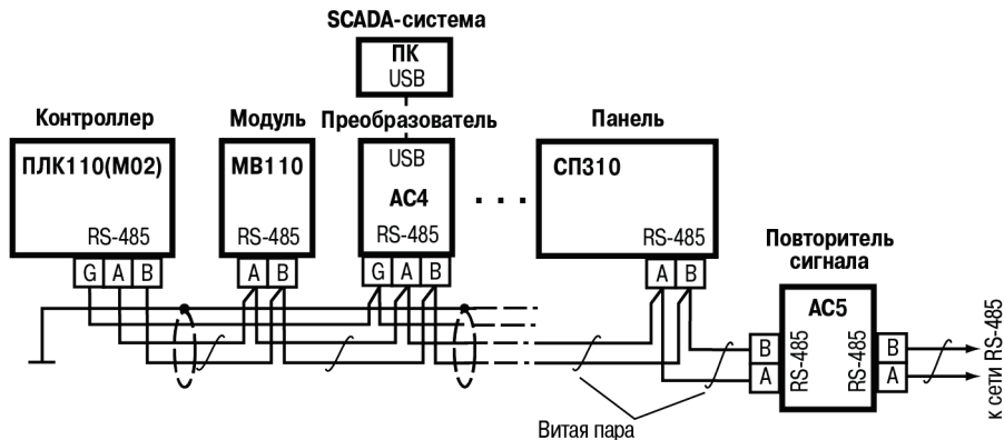
Рисунок 6.3 – Пример схемы подключения в сеть ПЛК110(M02) с другими приборами ОВЕН
