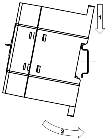
Рисунок 6.1 – Монтаж контроллера с креплением на DIN-рейку
