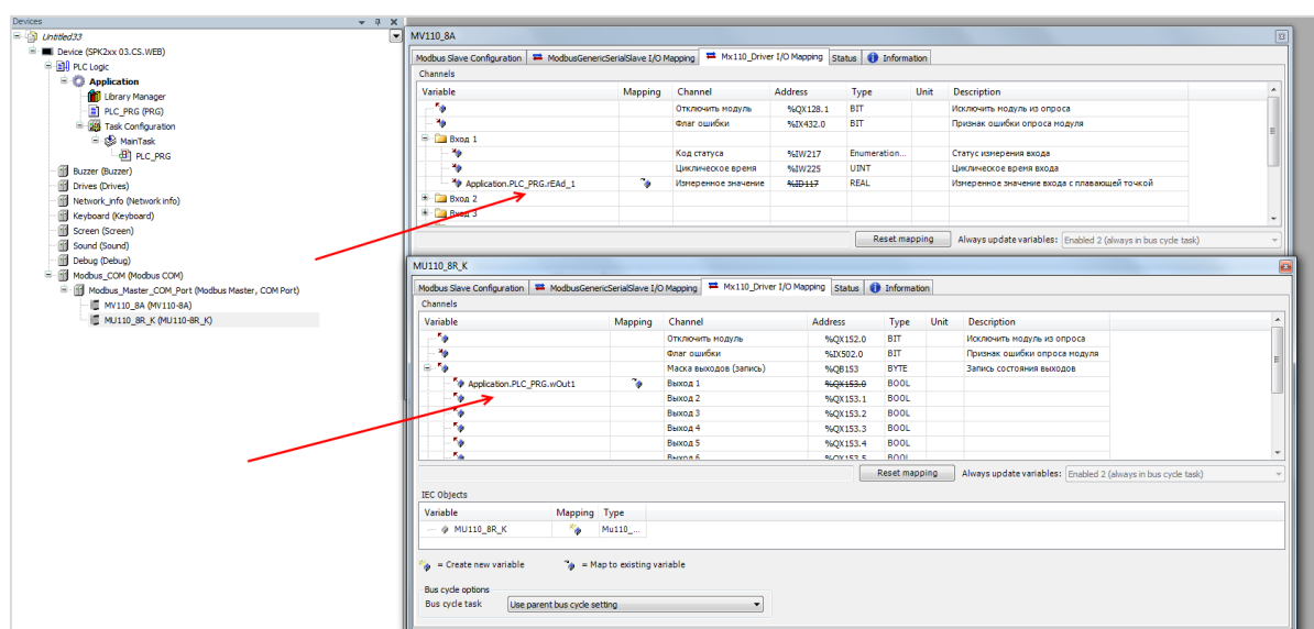
Рисунок 2.8 – Настройка шаблонов в среде CODESYS V3.5 SP11 Patch 5
