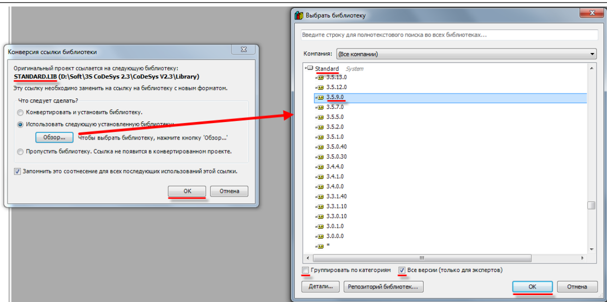
Рисунок 3.2 – Конверсия библиотек
