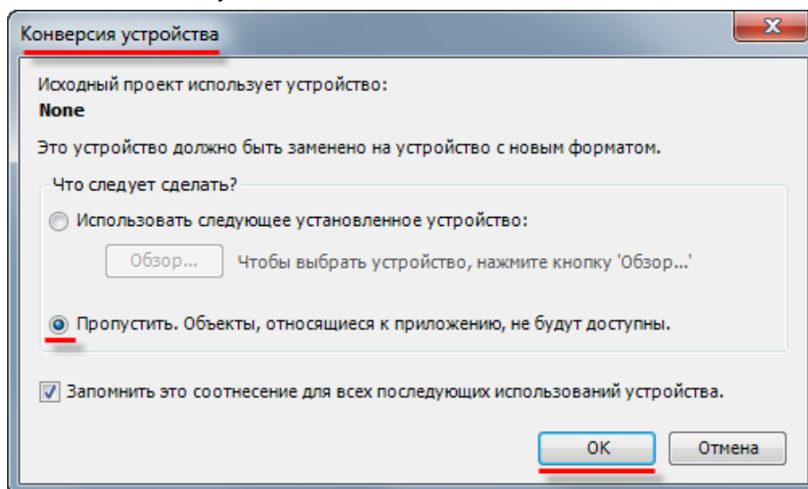
Рисунок 3.3 – Конверсия устройств
