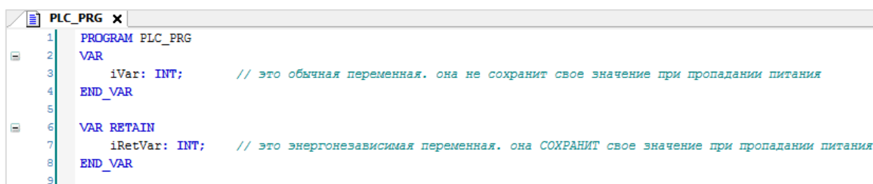
Рисунок 7.30 – Объявление энергонезависимых переменных
