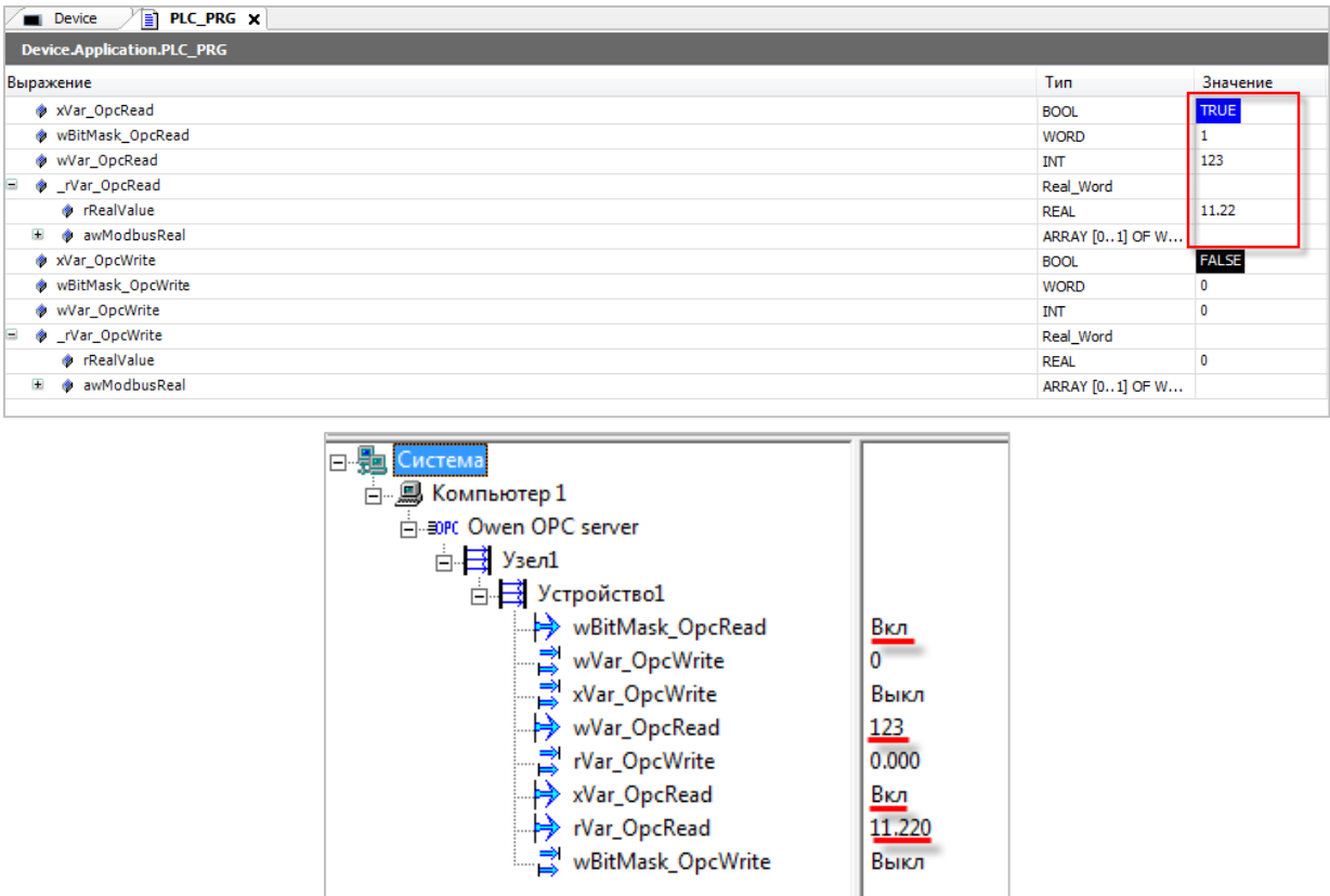
Рисунок 4.7.6 – Считывание данных из контроллера в MasterSCADA
