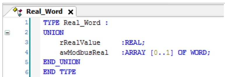
Рисунок А.2 – Объявление переменных объединения
