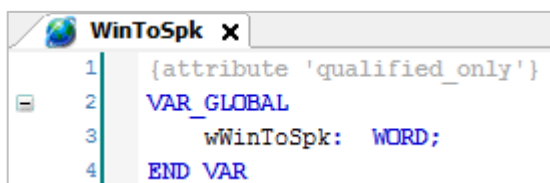
Рисунок 3.27 – Объявление отправляемых сетевых переменных для СПК1хх [M01]
