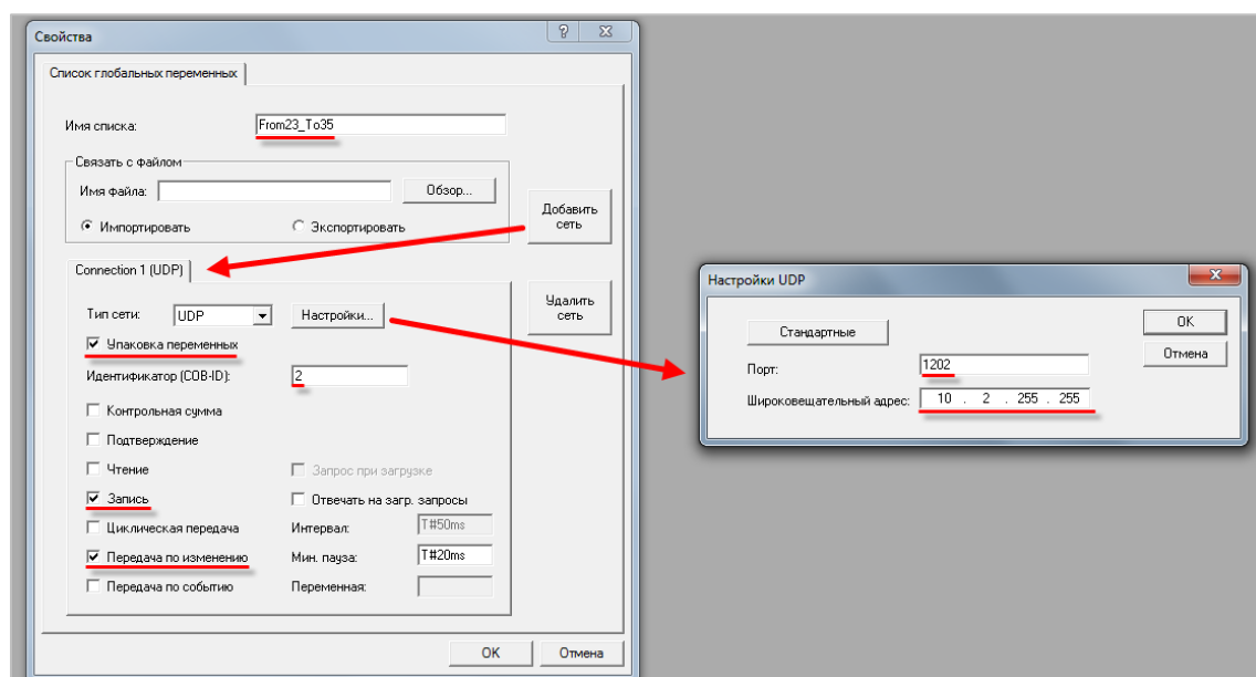
Рисунок 3.12 – Настройки списка отправляемых сетевых переменных для ПЛК110 [M02]
