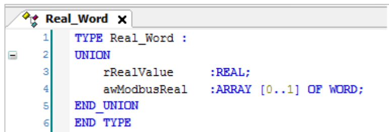
Рисунок 4.3.2 – Объявление переменных объединения
