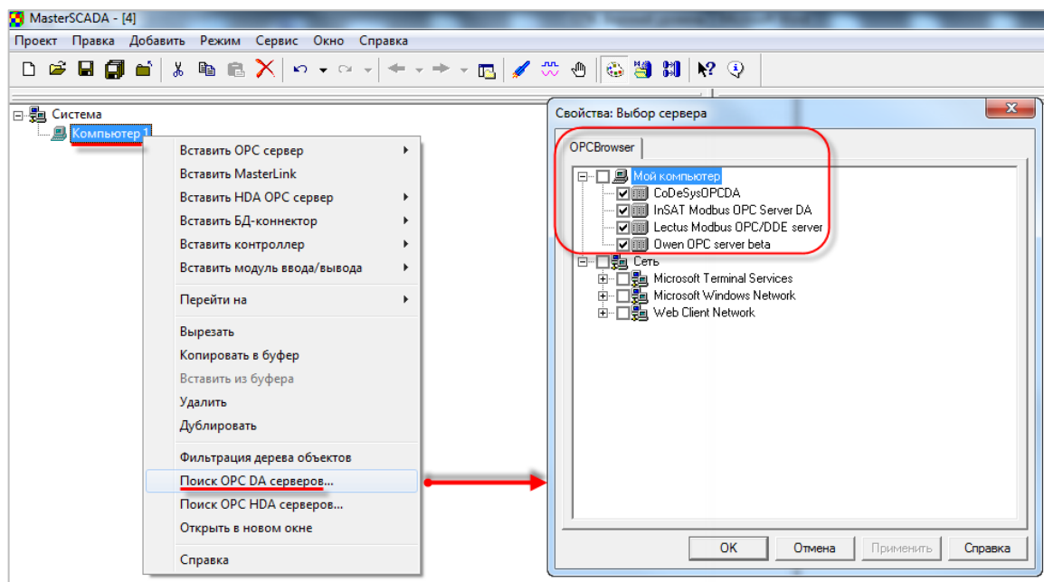
Рисунок 4.7.3 – Поиск установленных OPC-серверов
