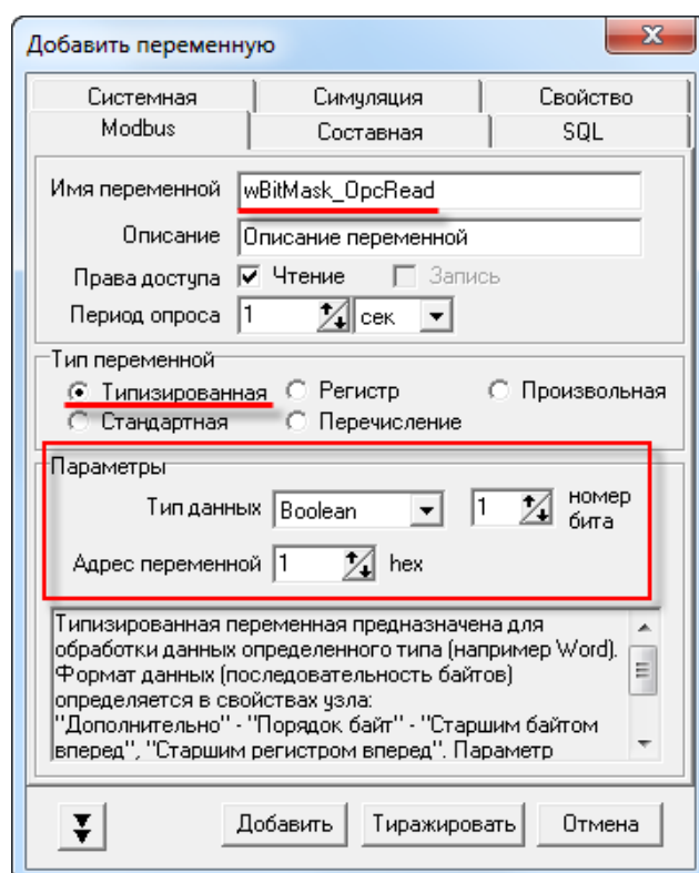
Рисунок 4.4.3 – Добавление и настройка переменной wBitMask_OpcRead
