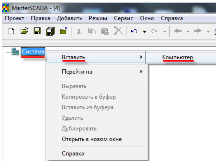
Рисунок 4.7.1 – Добавление узла Компьютер
