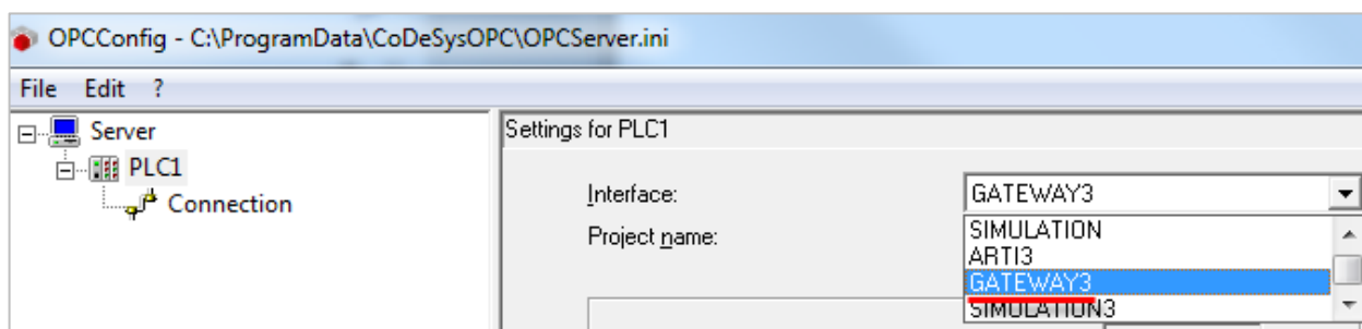
Рисунок 4.2.7 – Выбор интерфейса связи контроллера и OPC-сервера
