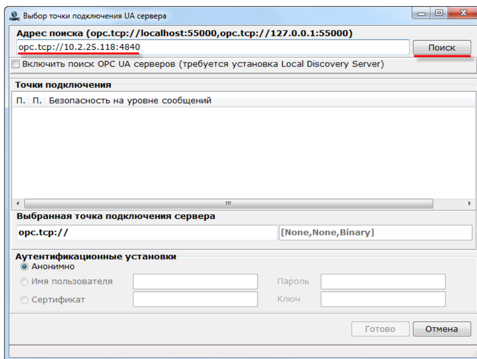
Рисунок 4.6.4 – Указание сетевых настроек OPC UA сервера
