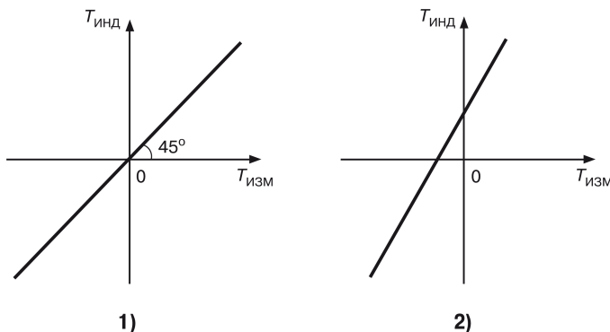
Рисунок 7.12 – Характеристики датчика: 1) исправного; 2) с погрешностями
