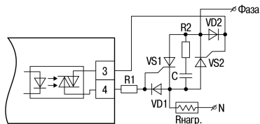
Рисунок 5.6 – Схема подключения двух встречно-параллельно включенных тиристорov к ВУ типа С
