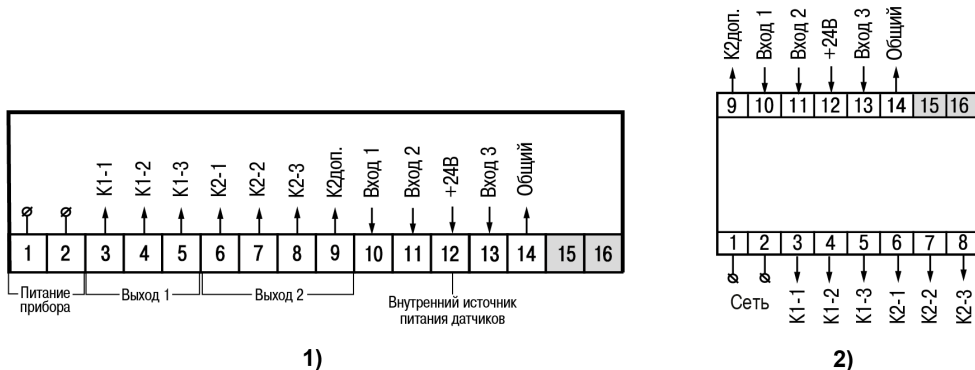
Рисунок 5.1 – Назначение контактов клеммника приборов настенного Н, щитового Щ1, Щ2 (1) и DIN-реечного (2) креплений
