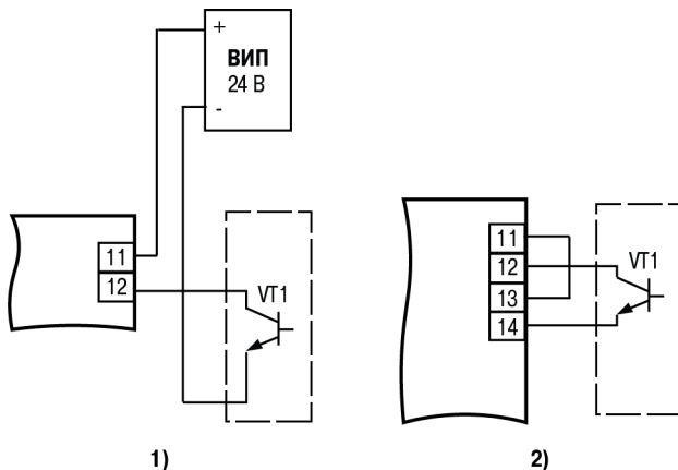
Рисунок 5.3 – Подключение пассивных датчиков с п-р-п-выходом: 1) при работе датчика от ВИП; 2) при работе датчика от внутреннего источника питания
