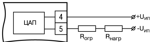
Рисунок 5.4 – Схема подключения ВУ типа И
