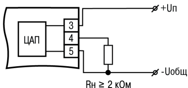
Рисунок 5.5 – Схема подключения ВУ типа У
