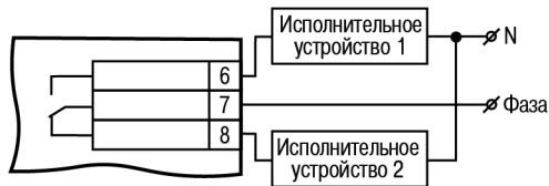
Рисунок 5.6 – Схема подключения нагрузки к ВУ типа Р
