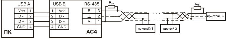
Рисунок 6.1 – Схема підключення
