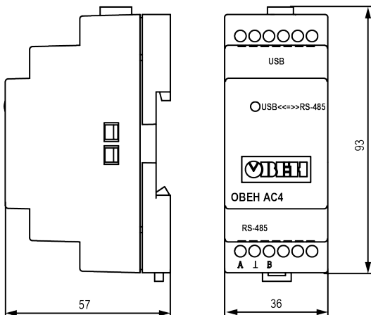
Рисунок 2.1 – Габаритні розміри
