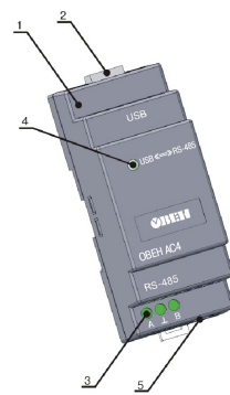
Рисунок 4.1 – Побудова пристрою
