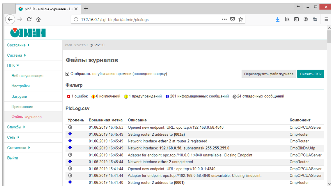
Рисунок 5-15: Страница «Файлы журналов»
