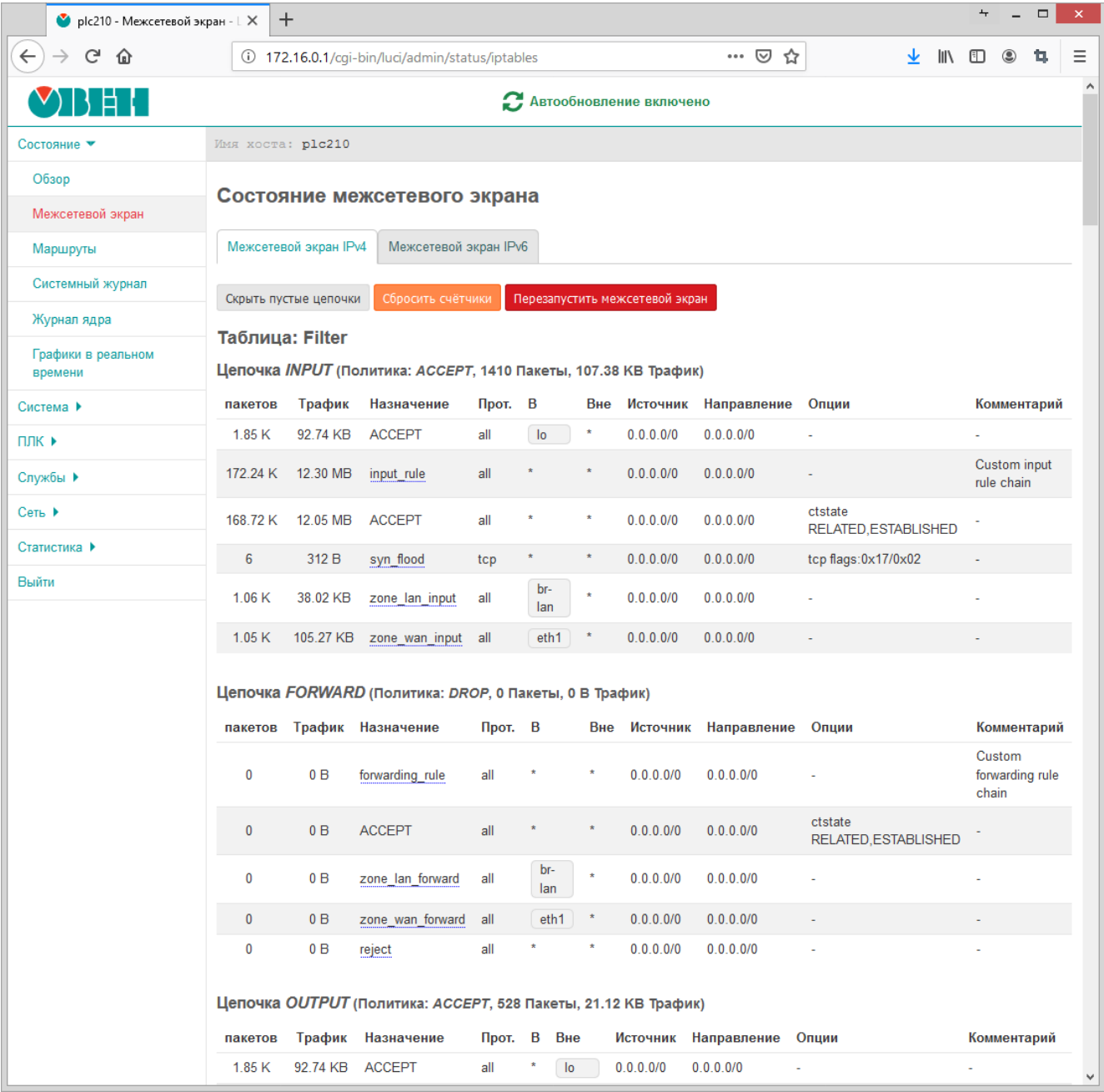
Рисунок 3-11: Страница «Межсетевой экран»
