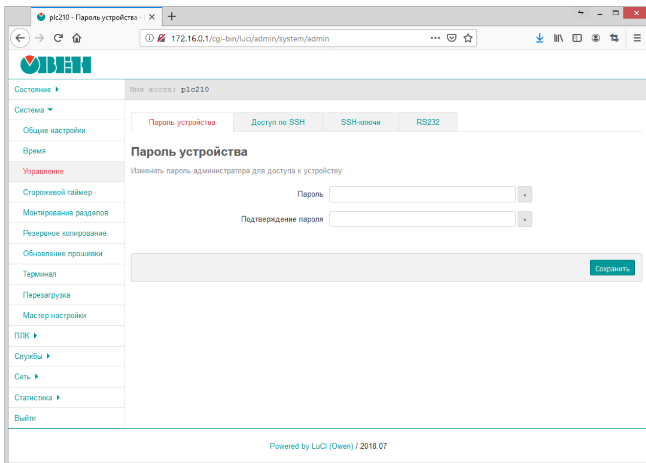
Рисунок 4-7: Страница «Управление». Вкладка «Пароль маршрутизатора»
