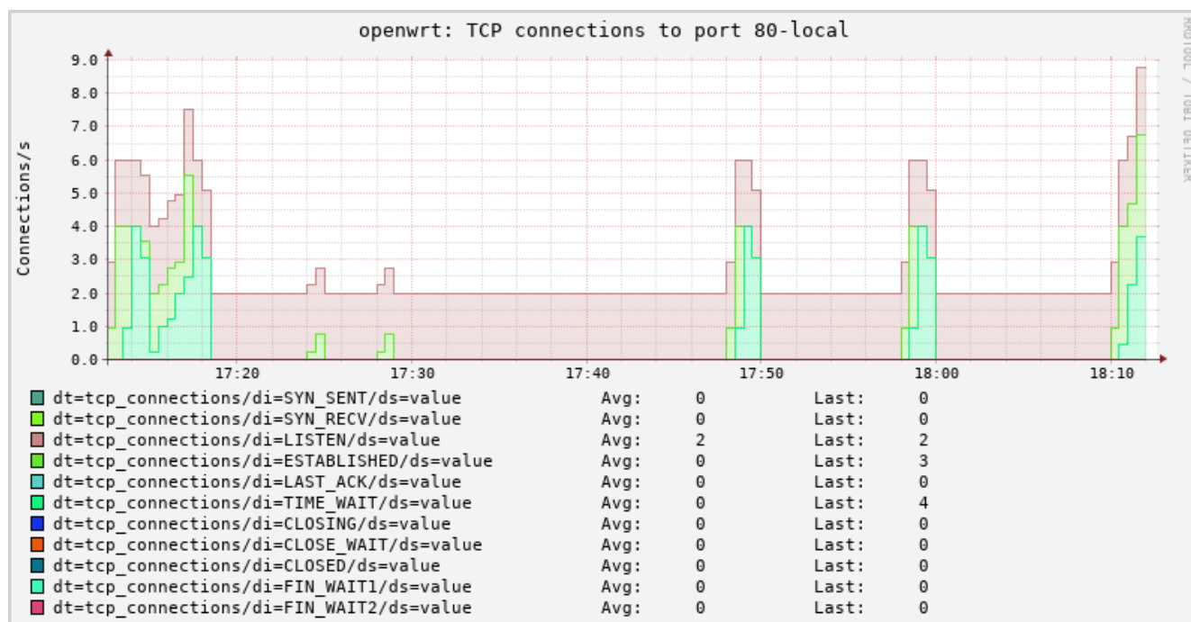
Рисунок 8-18: Статистика. График открытых соединений для TCP порта
