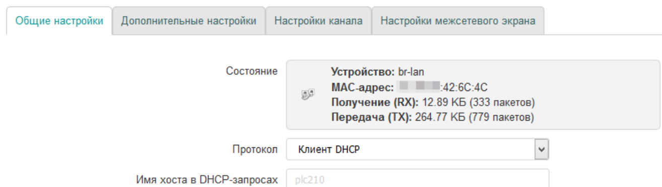
Рисунок 7-4: Общие настройки сетевого интерфейса
