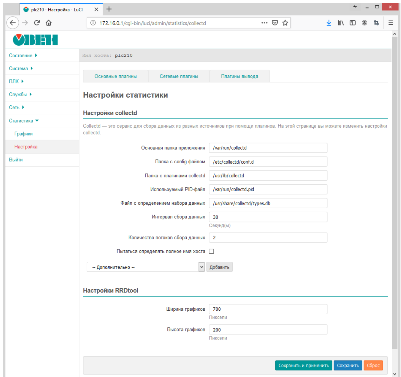
Рисунок 8-2: Настройки сбора и отображения статистики
