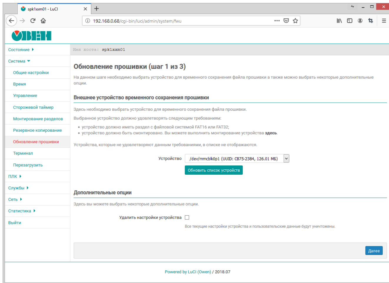
Рисунок 4-20: Страница «Обновление прошивки»
