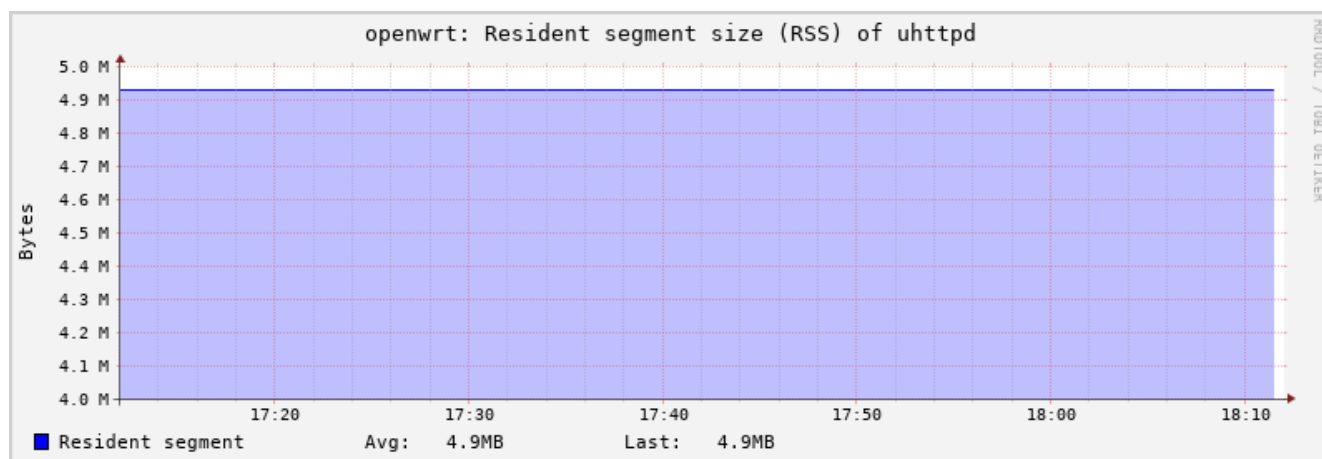
Рисунок 8-11: Статистика. График RSS процесса
