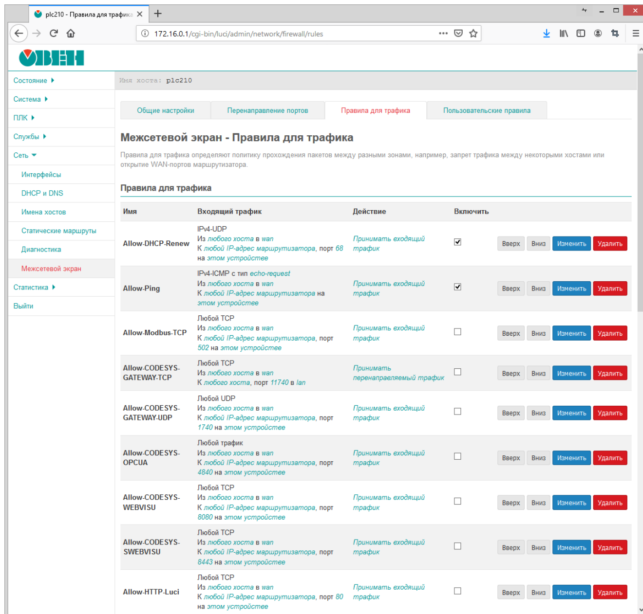
Рисунок 7-37: Правила для трафика межсетевого экрана
