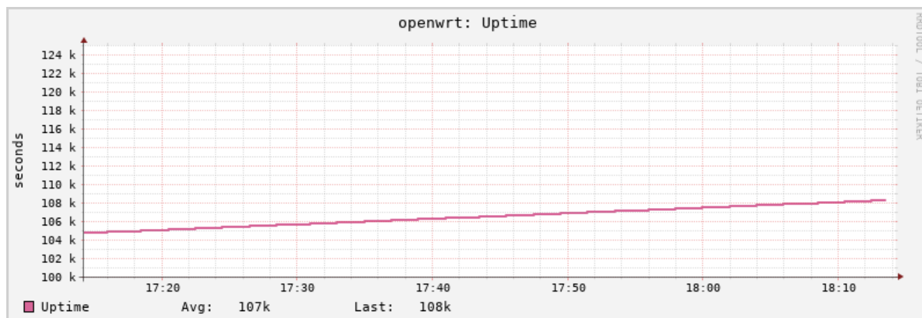
Рисунок 8-13: Статистика. График времени работы
