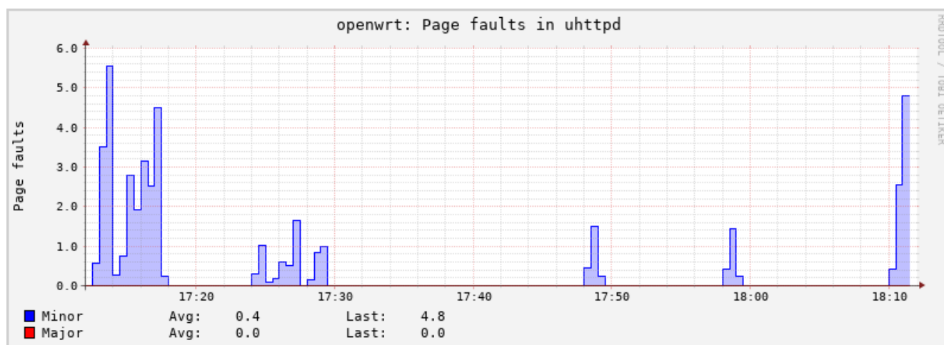
Рисунок 8-10: Статистика. График ошибок страниц процесса
