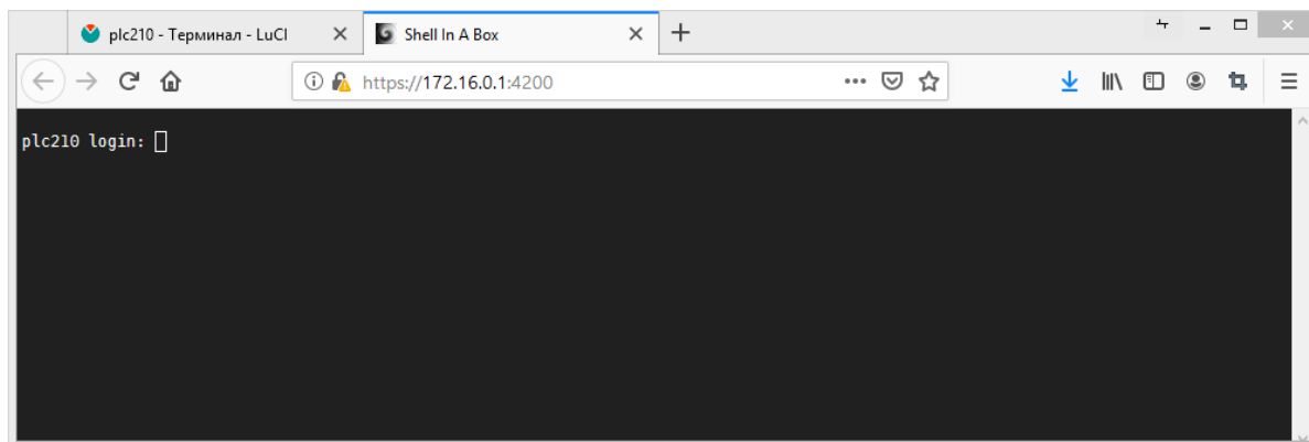
Рисунок 4-32: Страница «Терминал». Открытие терминала после подтверждения самоподписанного сертификата
