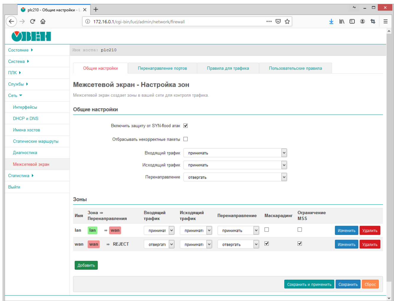
Рисунок 7-30: Общие настройки межсетевого экрана
