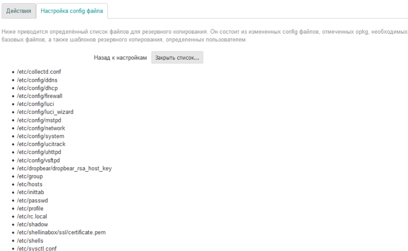
Рисунок 4-19: Страница «Резервное копирование». Вкладка «Настройка config файла». Список файлов
