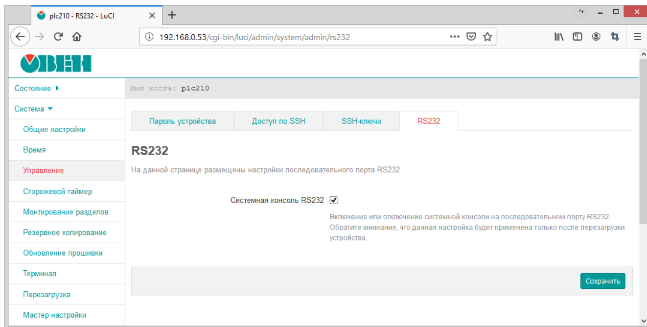
Рисунок 4-10: Страница «Управление». Вкладка «RS232»
