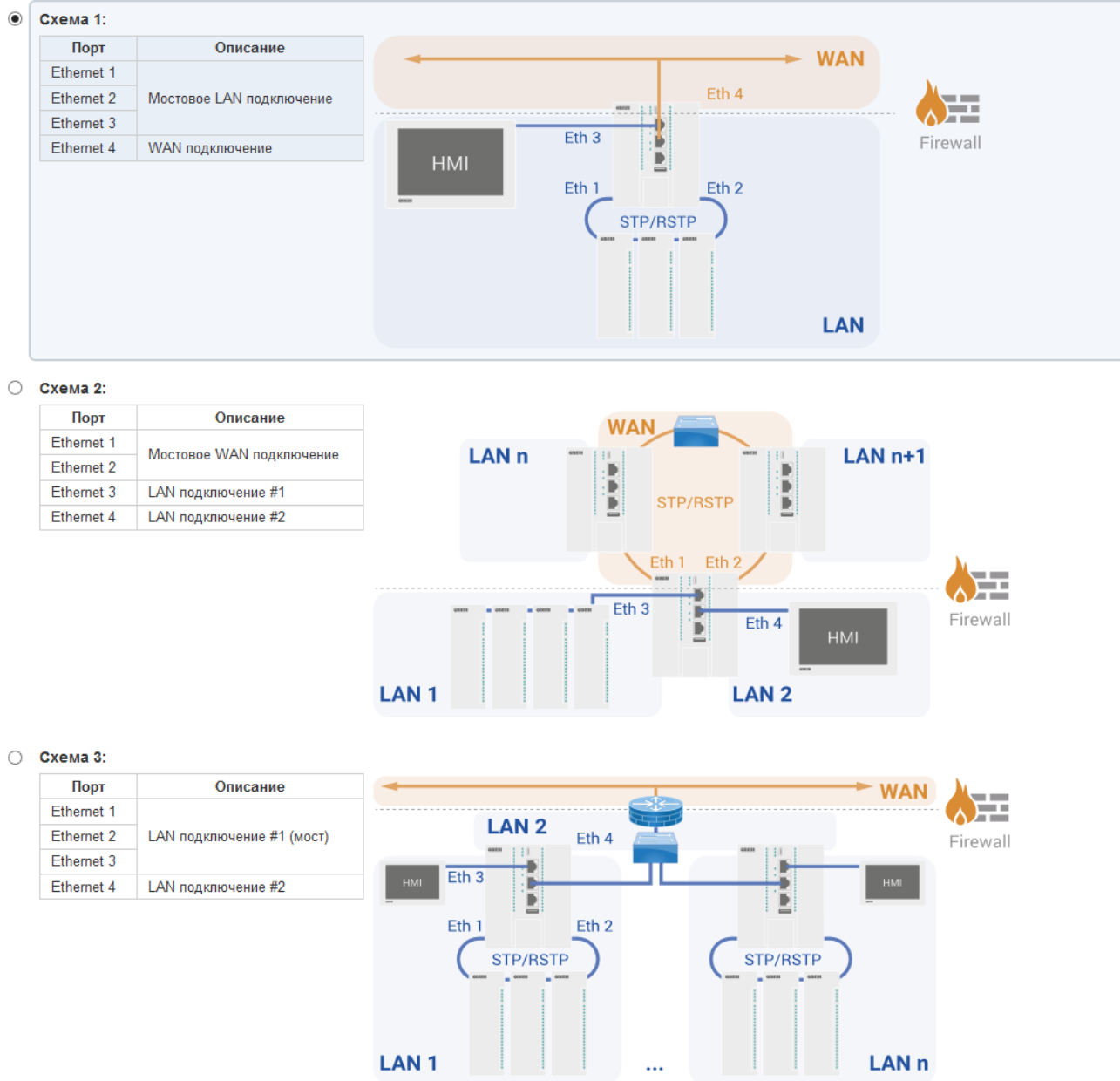
Рисунок 2-7: Мастер настройки. Выбор схемы сетевых портов
