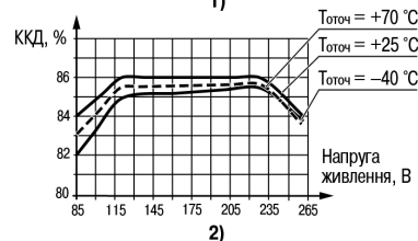
Рисунок 7 - Графік залежності ККД від напруги живлення і температури навколишнього середовища: (1) БП60А-12С, (2) БП60А-24С
