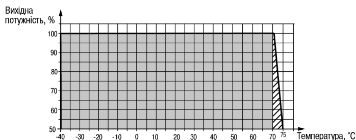
Рисунок 4 - Графік залежності вихідної потужності від температури навколишнього середовища
