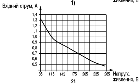
Рисунок 6 - Графік залежності вхідного струму від напруги живлення: (1) БП60А-12С, (2) БП60А-24С
