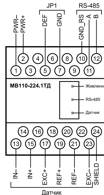
Рисунок 1 – Назначение контактов клеммника
