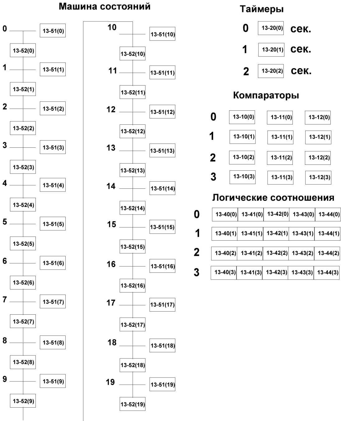
Рисунок 4.21 – Встроенный ПЛК ПЧВ1,2
