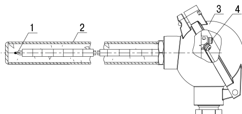
Рисунок 3.1 – Конструкция датчика с коммутационной головкой
