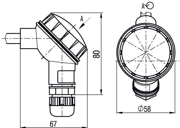
Рисунок Г.1 – Габаритные размеры пластмассовой коммутационной головки
