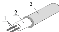
Рисунок 3.3 – Конструкция ЧЭ на основе КТМС
