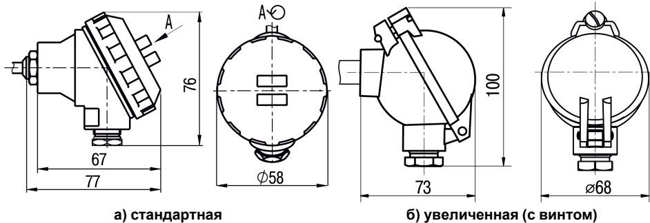
Рисунок Г.2 – Габаритные размеры металлической коммутационной головки
