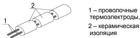
Рисунок 3.2 – Конструкция проволочного ЧЭ
