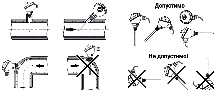
Рисунок 5.3 – Монтаж датчика с коммутационной головкой
