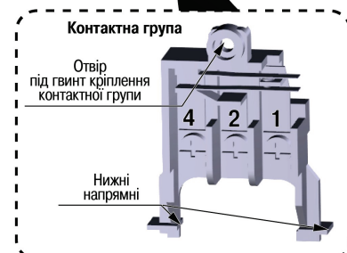
Рисунок 4.2 – Будова пристрою
