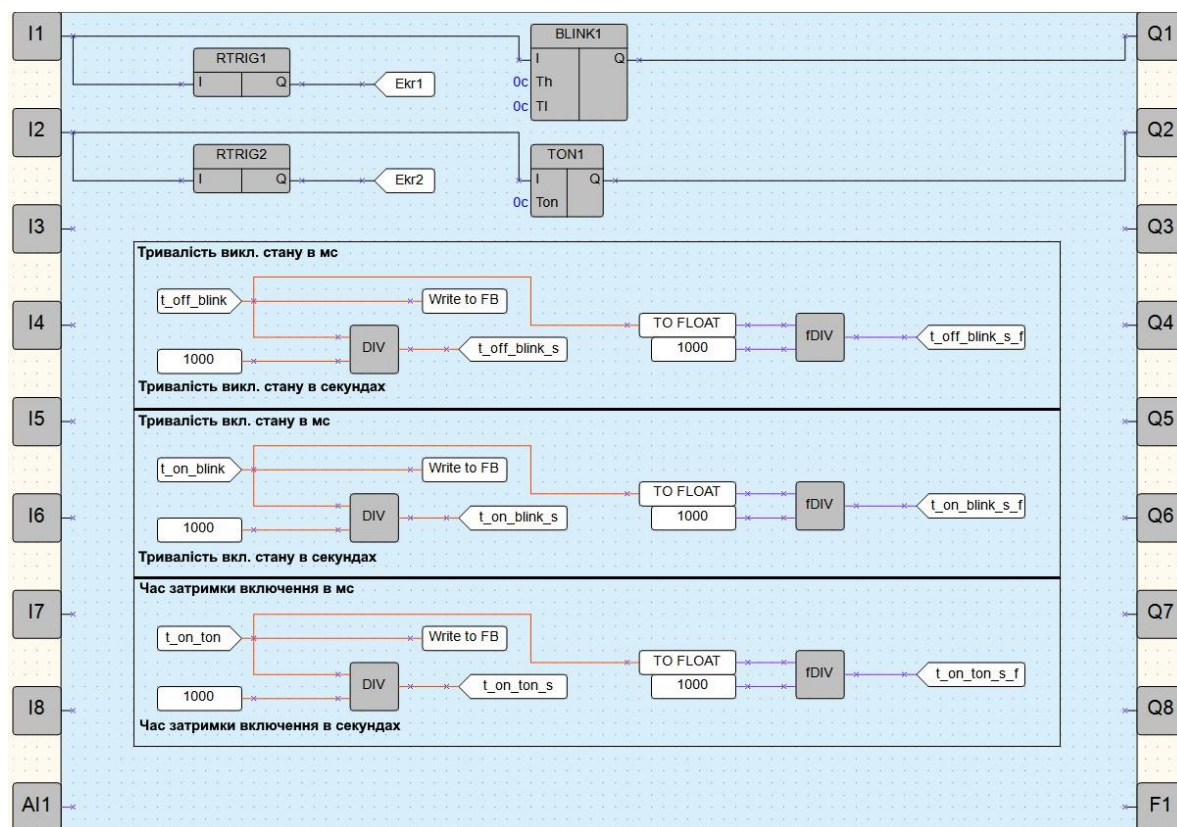
Рисунок 10.11 – Схема алгоритму
