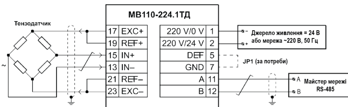
Рисунок 5.4 – Підключення до пристрою MB110-224.1TD зовнішніх пристроїв за допомогою чотирипроводової схеми підключення до датчика та за допомогою заземлення
