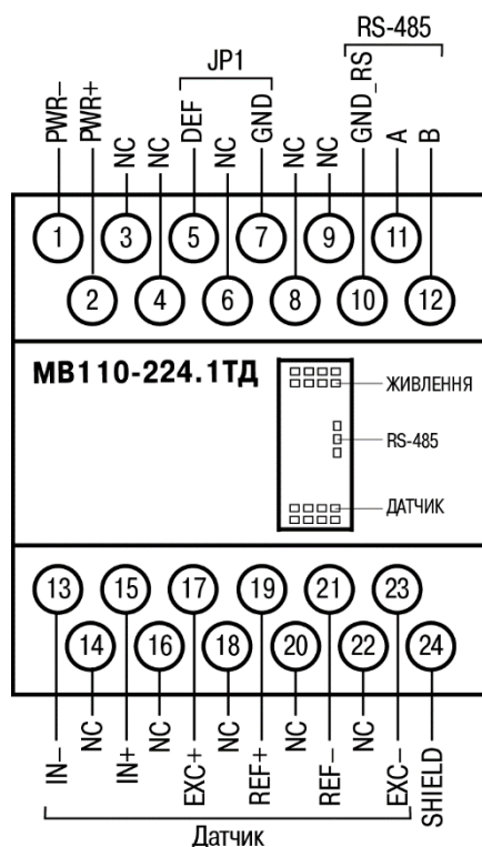
Рисунок 5.2 – Призначення контактів клемної колодки MB110-224.1ТД
