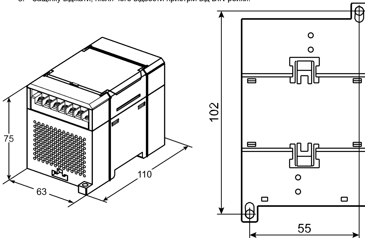
Рисунок 4.1. – Габаритні та установчі розміри
