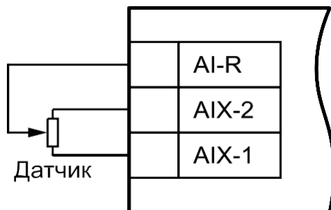
Рисунок 5.8. – Схема підключення датчика положення резистивного типу 0...5000 Ом
