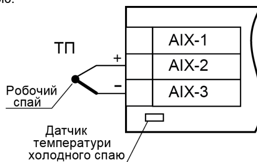
Рисунок 5.4 – Схема підключення ТП
