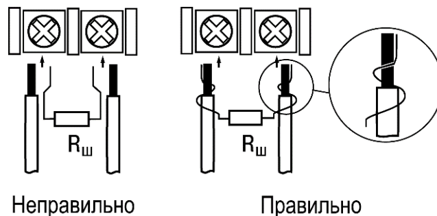
Рисунок 5.7 – Підключення шунтувального резистора
