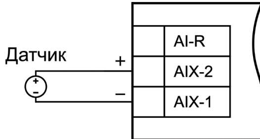
Рисунок 5.5 – Схема підключення активного датчика з виходом у вигляді напруги -50...50 мВ або 0...1 В
